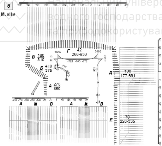
Рис.3. Результати розрахунків 3D моделі: епюри горизонтальних переміщень (U) та згинальних моментів (M) у палях підірної стіни огороження котловану (приклад 1)
