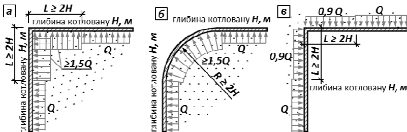
Рис. 1. Принципові схеми урахування форми споруди для визначення навантажень від тиску ґрунту на підпiрну споруду
