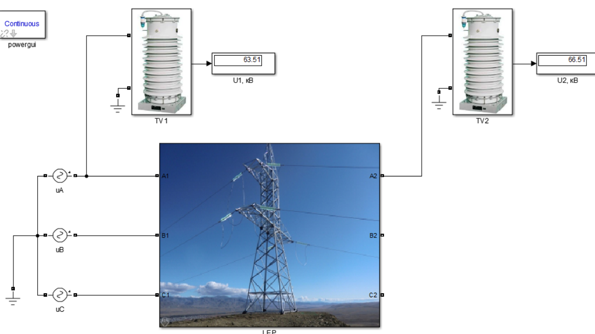
Рис. 4.19. Схема віртуальної лабораторної установки
