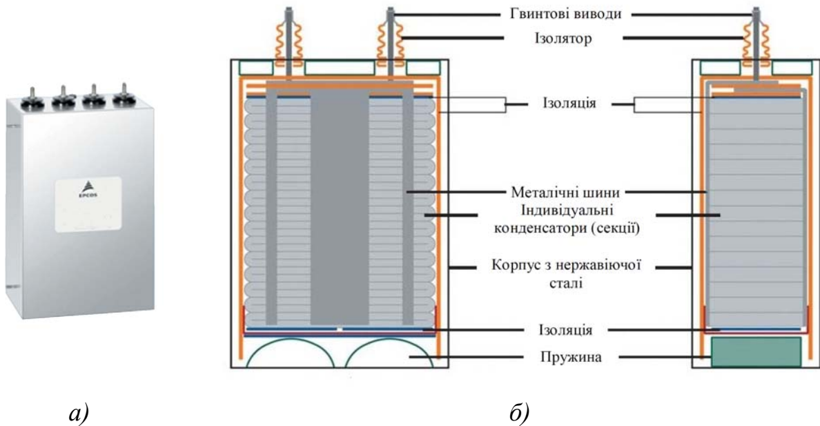
Рис. 3.14. Силовий оливнаповнений конденсатор МКК DCI від EPCOS: а – загальний вигляд; б – конструкція
