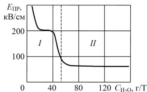
Рис. 1.27. Залежність електричної міцності трансформаторної оливи від вмісту вологи, C_{H_2O} (грам/тона): I – зона розчинення вологи; II – емульгована волога
