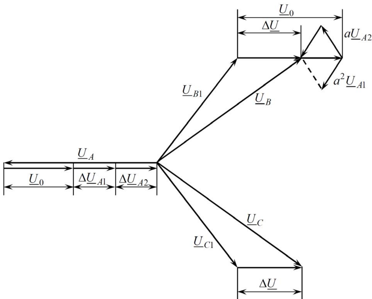
Рис. 2.42. Векторна діаграма напруг при однофазному КЗ
