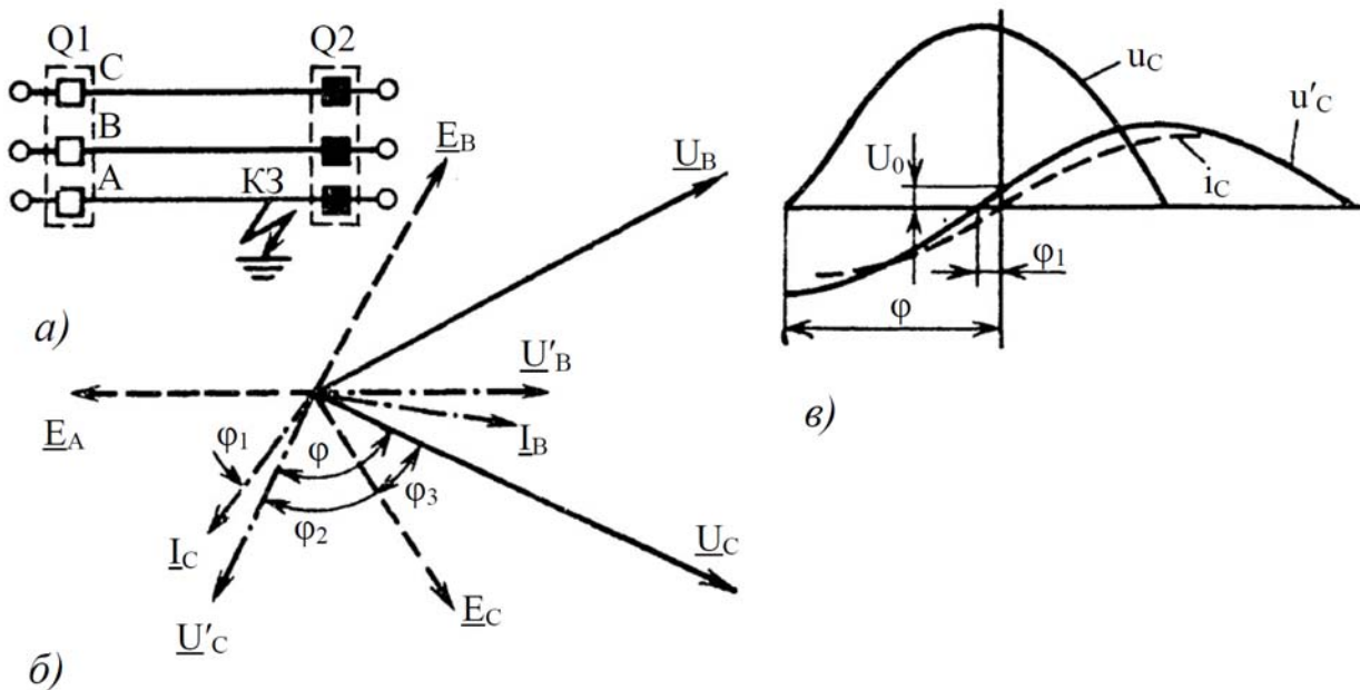
Рис. 2.29. Відключення однофазного КЗ: а – розрахункова схема; б – векторна діаграма струмів і напруг; в – криві напруги в місці КЗ до і після відключення
