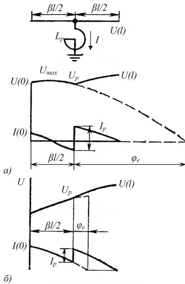
Рис. 2.40. Розподіл напруги і струму в односторонньо включеній лінії з реактором в середині лінії: a – при великій потужності реактора; б – при малій потужності реактора
