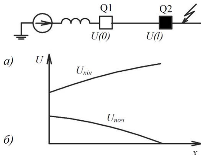
Рис. 2.27. Відключенні струму КЗ: а – схема; б – розподілення напруги до відключення ( U_{поч} ) і після відключення ( U_{кін} )
