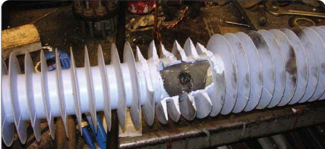
Рис. 1.8. Пропалювання та пробій полімерного ізолятора на роз'єднувачі 110 кВ
