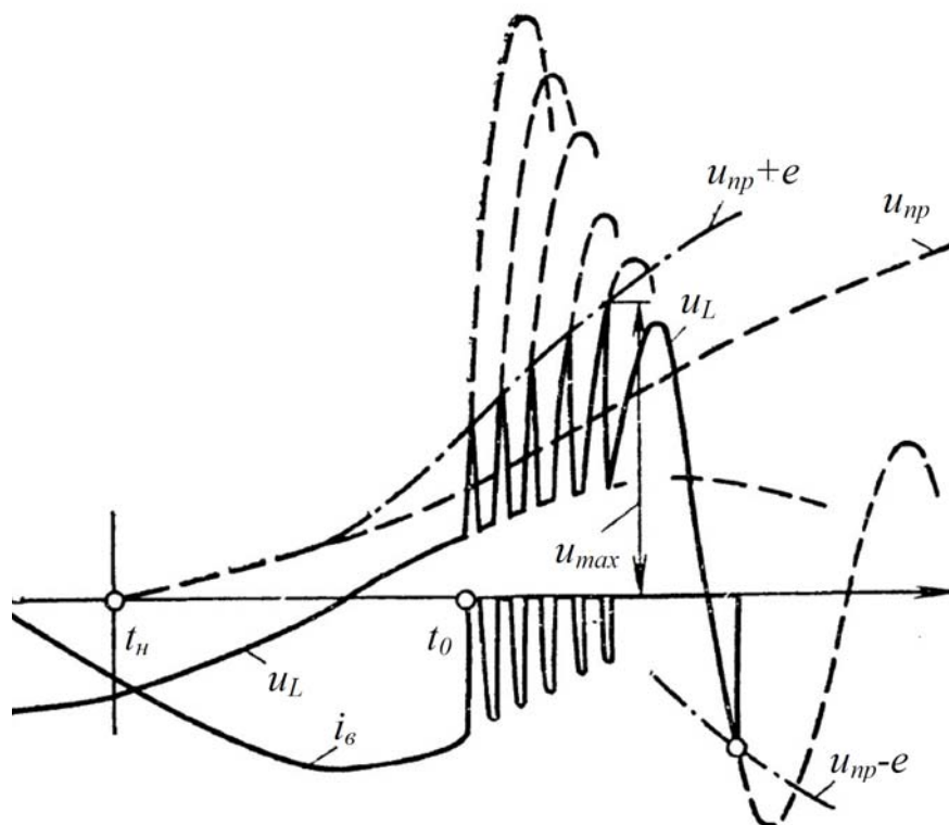
Рис. 2.32. Перехідний процес при відключенні ненавантаженого трансформатора
