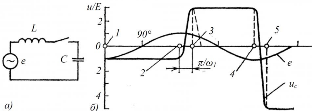
Рис. 2.23. Напруга на ємності при повторних запалюваннях дуги у вимикачі: а – розрахункова схема; б – криві напруги перехідного процесу при запаленні дуги в моменти проходження ЕРС через максимум
