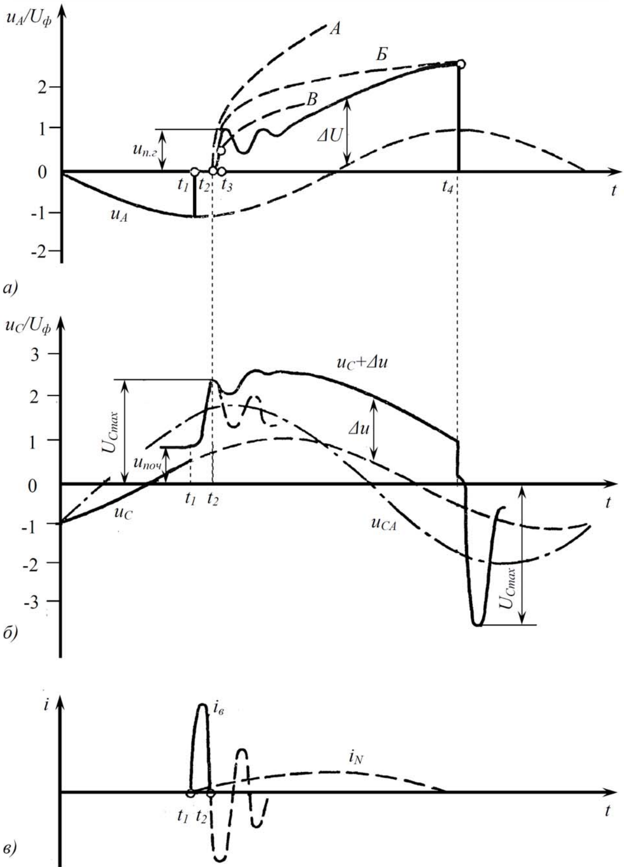
Рис. 2.34. Напряга переходного процесу при дуговому КЗ: а – напруга фази А; б – напруга фази С; в – струм в місці замикання
