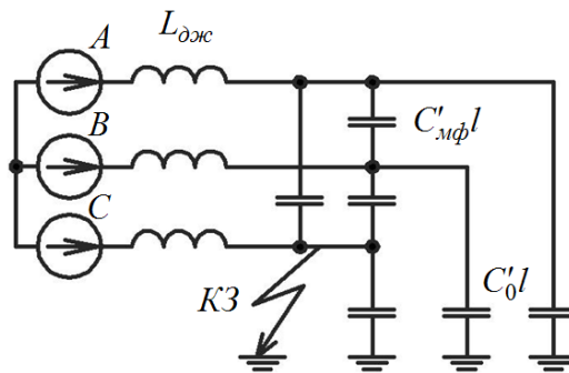
Рис. 2.33. Схема заміщення мережі з ізолюваною нейтраллю: C'_0 – ємність фази на землю; C'_{mf} – міжфазна ємність; L_{дж} – індуктивність джерела
