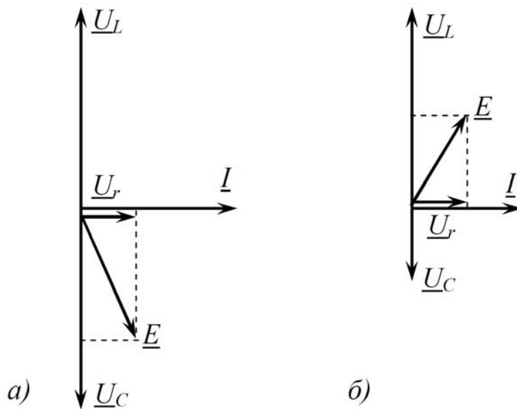
Рис. 2.48. Векторні діаграми для ферорезонансного контуру: а – емнісний режим; б – індуктивний режим
