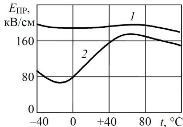
Рис. 1.30. Залежність електричної міцності трансформаторної оливи від температури: 1 – суха олива; 2 – технічна олива з домішкою вологи
