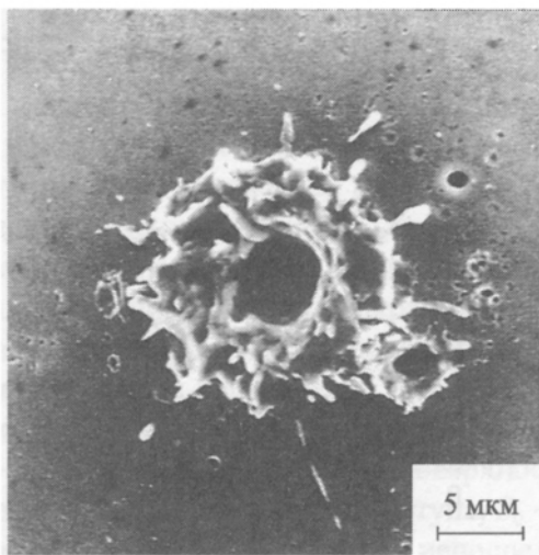
Рис. 1.22. Знімок поверхні плоского мідного катода після однократного ввімкнення струму при довжині імпульсу 20 нс
