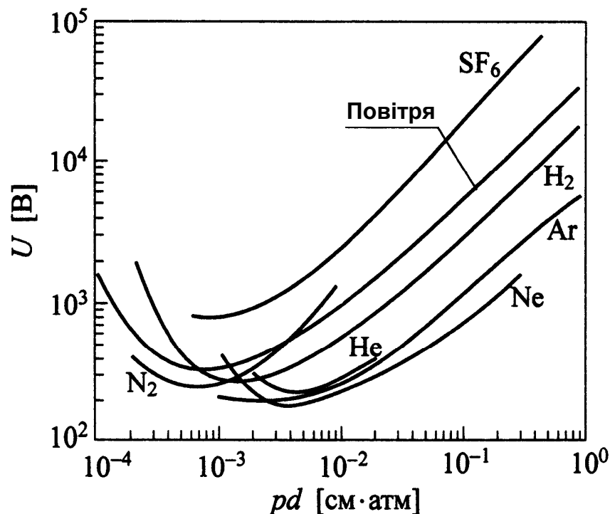
Рис. 1.24. Залежність напруги пробую від величини pd для різних газів (криві Пашена)
