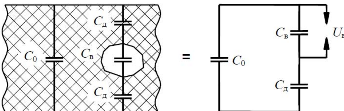
Рис. 1.37. Схема заміщення твердого діелектрика: C_0 – ємність бездефектної ізоляції; C_g – ємність повітряного включення; C_d – ємність діелектрика послідовно з включенням; U_g – напруга пробою повітряного включення
