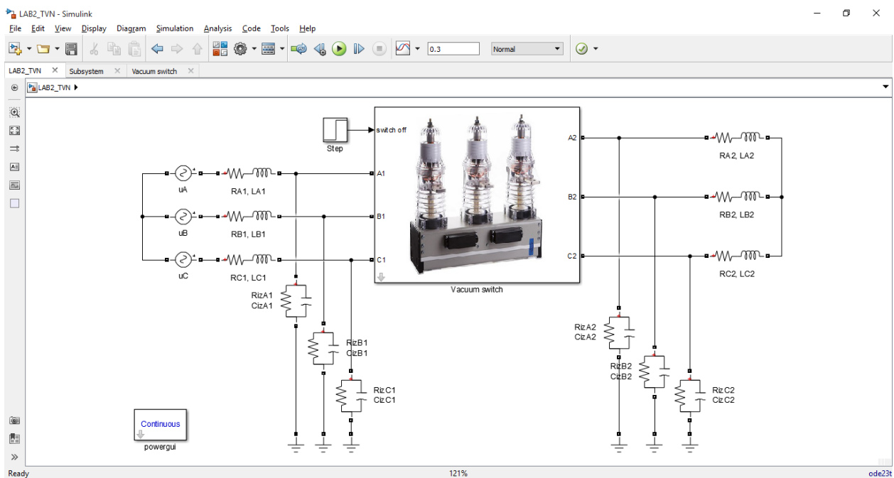
Рис. 4.5. Загальний вигляд віртуального лабораторного стенда у програмі Simulink (файл LAB2_TVN.slx)
