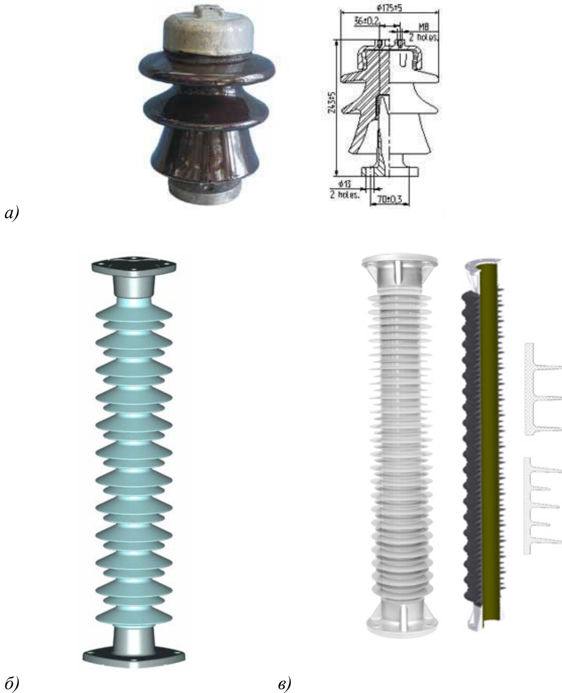
Рис. 3.6. Опорні ізолятори зовнішнього встановлення: а – опорний штировий ізолятор ОНШ-15-5; б – опорний стержневий кремнійорганічний ізолятор ОСК 10-110-А01-2; в – опорний порожнинний полімерний ізолятор
