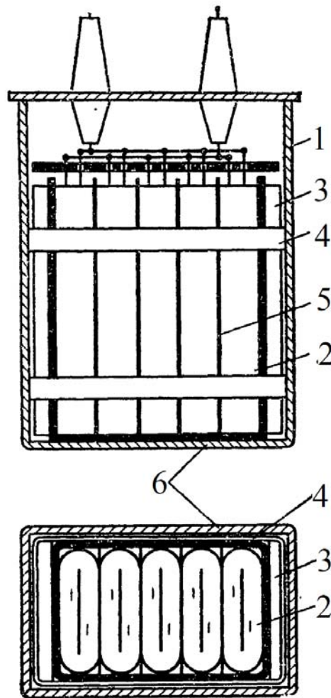
Рис. 3.13. Схематична конструкція силового конденсатора для підвищення коефіцієнта потужності: 1 – герметизований корпус; 2 – рулонні секції; 3 – металічні щоки; 4 – хомут; 5 – ізолююча прокладка; 6 – ізоляція від корпусу
