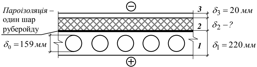
Рис. 7. Розрахункова схема горищного перекриття
