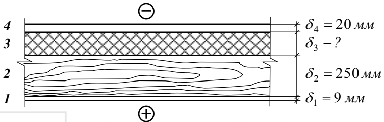
Рис. 5. Розрахункова схема конструкції горіщного перекриття (переріз 1-1)
