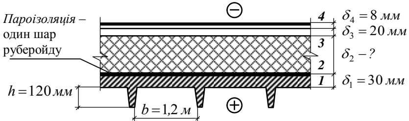
Рис. 8. Розрахункова схема покриття
