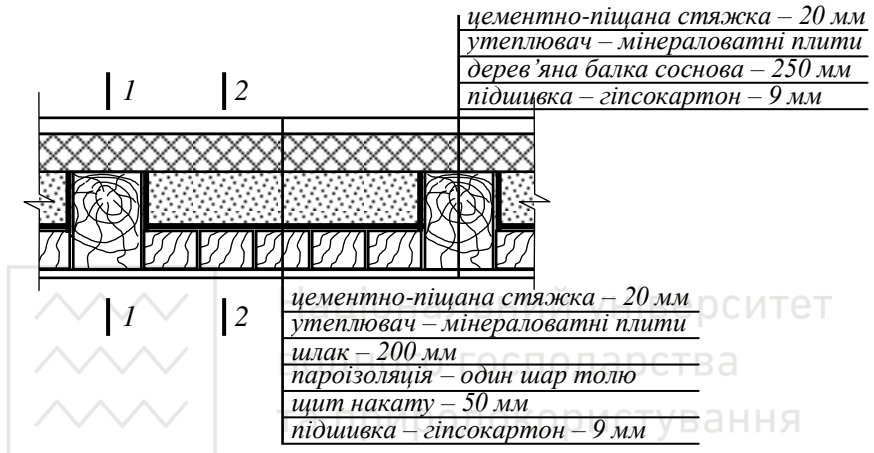
Рис. 4. Конструкція горищного перекриття
