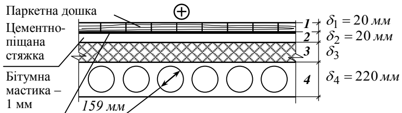
Рис. 9. Розрахункова схема конструкції перекриття над підвалом
