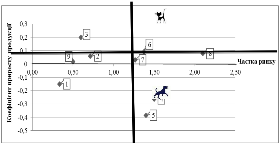
Рисунок 1 – Матриця БКГ
