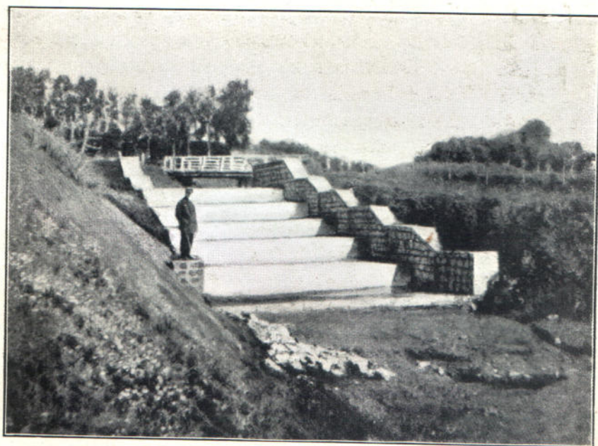
Каменно-бетонный водосливъ съ перепадами.
