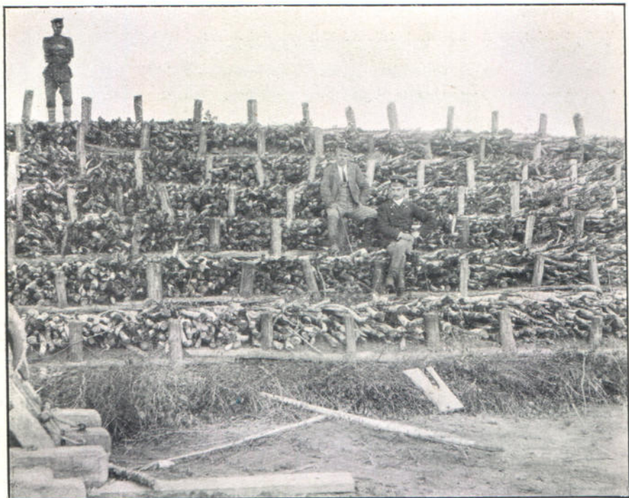
Укрѣпленіе берега хворостомъ.
