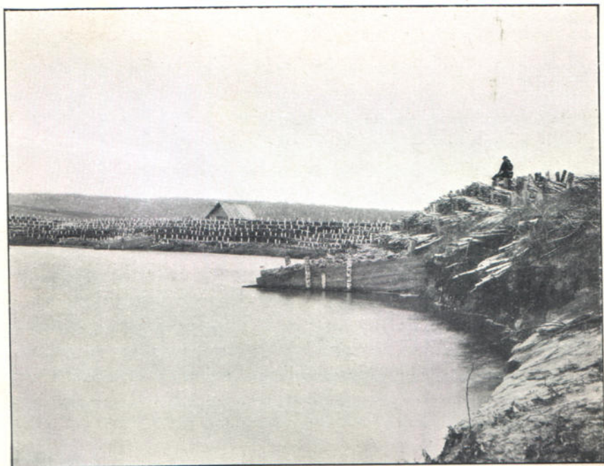
Общій видъ укрѣпленія берега хворостомъ.
