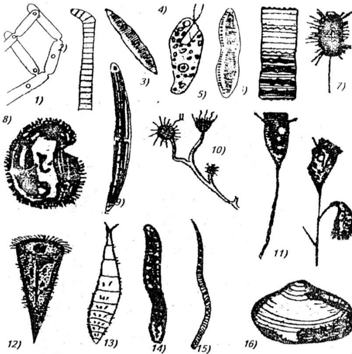
Мал. 2. Організми \alpha - мезосапробної зони: 1) - Leptomitus lacteus ; 2) - Oscillatoria formosa ; 3) - Nitzschia palea ; 4) - Chilomonas paramecium ; 5) - Nitzschia amphioxys ; 6) - Stephanodiscus hantzschii ; 7) - Uronema marinum ; 8) - Chilodonella uncinata ; 9) - Closterium acerosum ; 10) - Anthophysa vegetans ; 11) - Vorticella convallaria ; 12) - Stentor coeruleus ; 13) - Larve Stratiomys ; 14) - Spirostonum ambiguum ; 15) - Herpobrella atomapia ; 16) - Sphaerium corneum .
