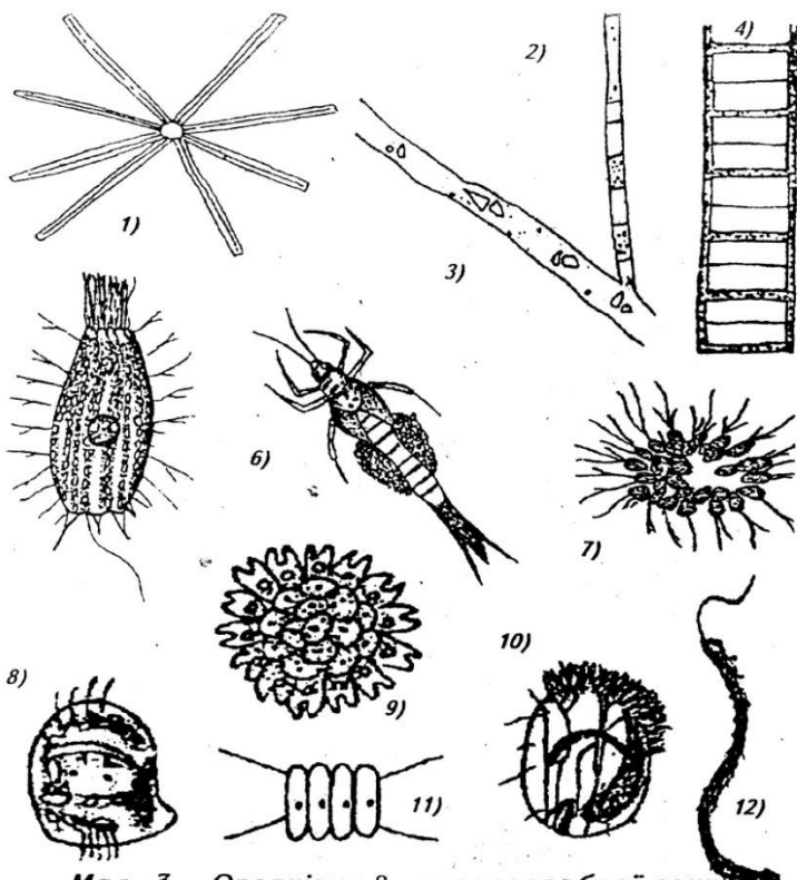
Мал. 3. Організми \beta - мезосапробної зони.
