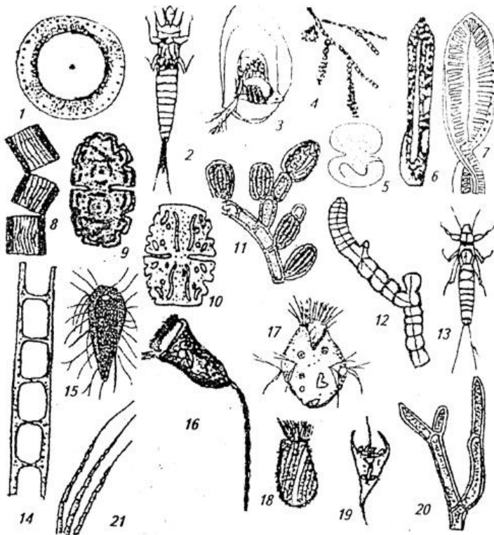
Мал. 4 . Організми олігосеєпробної зони:
