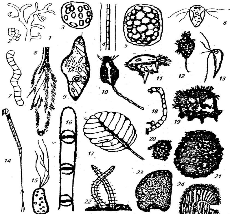
Мал. 1 . Організми полісапробної зони: 1 - Zoogloea ramigera ; 2 - Sarcina paludosa ; 3 - Chlorobacterium aggregatum ; 4 - Sphaerotilus natans ; 5 - Achromatium oxaliferum ; 6 - Trigonomonas compressa ; 7 - Spirulina jenniferi ; 8 - Sphaerotilus natans ; 9 - Euglena viridis ; 10 - Vorticella microstoma ; 11 - Caenomorpha medusula ; 12 - Trimyema compressa ; 13 - Tetramoria pyriformis ; 14 - Rotaria neptunia ; 15 - Chromatium okenii ; 16 - Oscillatoria putrida ; 17 - Lamprocystis roseopersicina ; 18 - Chironomus thummi ; 19 - Saprodinium dentatum ; 20 - Hexotricha caudata ; 21 - Glaucoma scintillans ; 22 - Tubifex rivulorum ; 23 - Pelomyxa palustris ; 24 - Paramaecium putrinum
