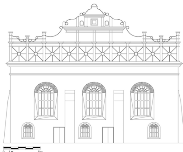
Рис. 5. Головний західний фасад. Опрацювання автора
