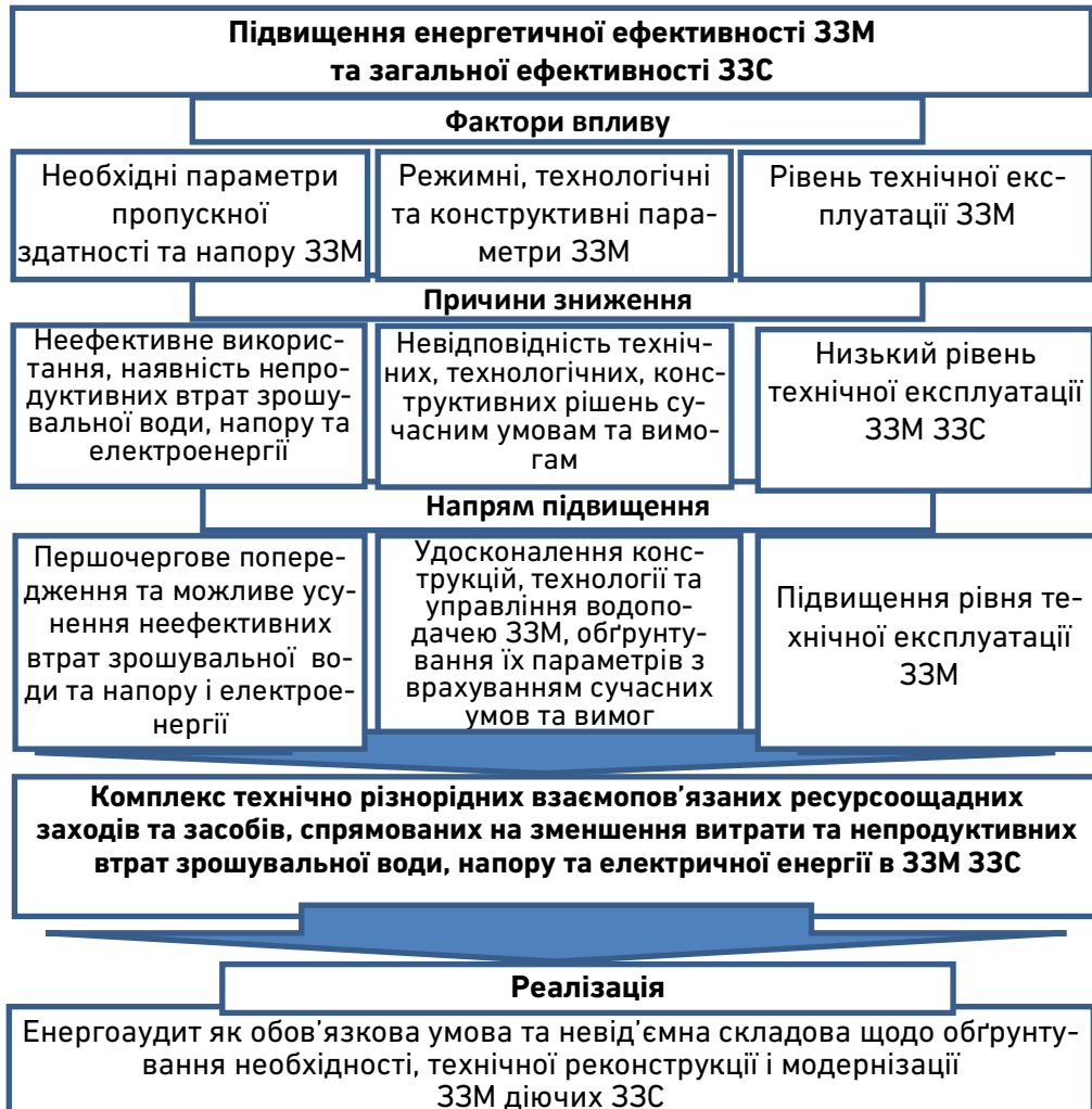
Рис. 2. Структурно-логічна схема підвищення енергетичної ефективності ЗЗМ та загальної ефективності ЗЗС за системною методологією
