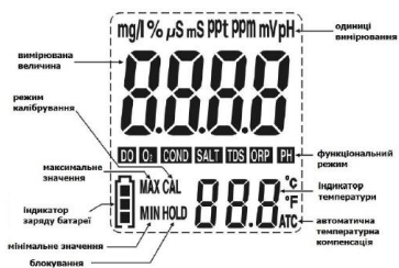
Рис. 4.1. Солемір Ezodo E7200: а) опис приладу; б) опис дисплея
