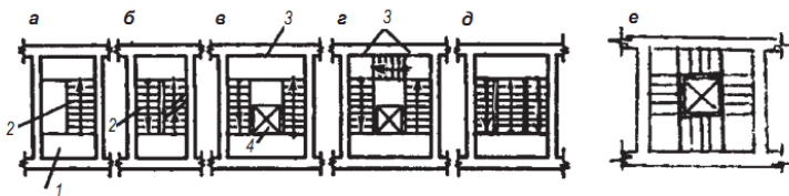
Рис. 10.2. Типи сходів: а – одномаршові; б, в – двомаршові; г, д – тримаршові; (в, г, е – сходи з ліфтами); е – чотиримаршові; 1 – поверхнева площадка; 2 – марш; 3 – сходові міжповерхові площадки; 4 – ліфт
