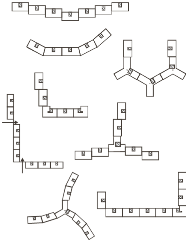
Рис. 3. Варіанти конфігурації житлових будинків з різних типів блок-секцій
