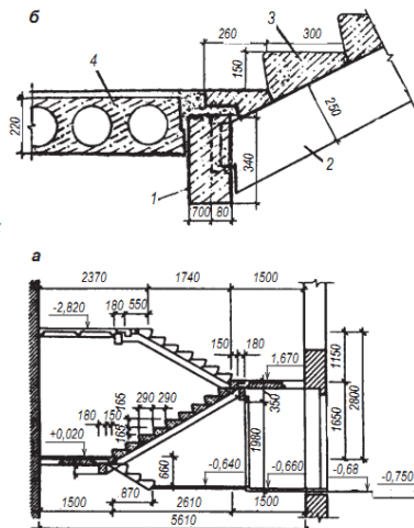
Рис. 10.5. Сходи зі збірних малорозмірних елементів: а – в розрізі; б – деталь сходів; 1 – площадкова балка; 2 – залізобетонний косоур; 3 – сходи; 4 – залізобетонна плита площадки
