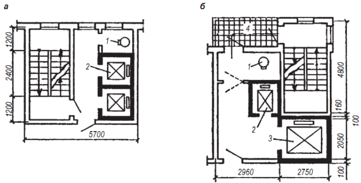
Рис. 10.3. Планувальні рішення сходів у будівлях підвищеної поверховості: а – захищені від диму й вогню ізольованими сходовими клітками; б – незадимлені; 1 – сміттепровід; 2 – пасажирський ліфт; 3 – вантажопасажирський ліфт; 4 – лоджія
