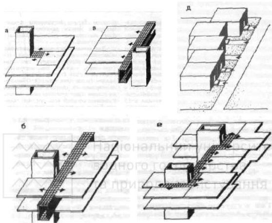
а) секційний; б) коридорний; в) галерейний; д) блоковий; е) змішаної структури
