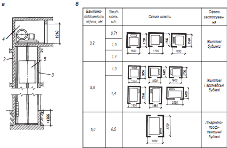
Рис. 20. Будівельні елементи ліфта та схеми шахти: а - будівельні елементи ліфта, б - схеми шахти, 1 - прямок, 2 - стінка шахти, 3 - двері шахти, 4 - машинне відділення, 5 - кабіна ліфта
