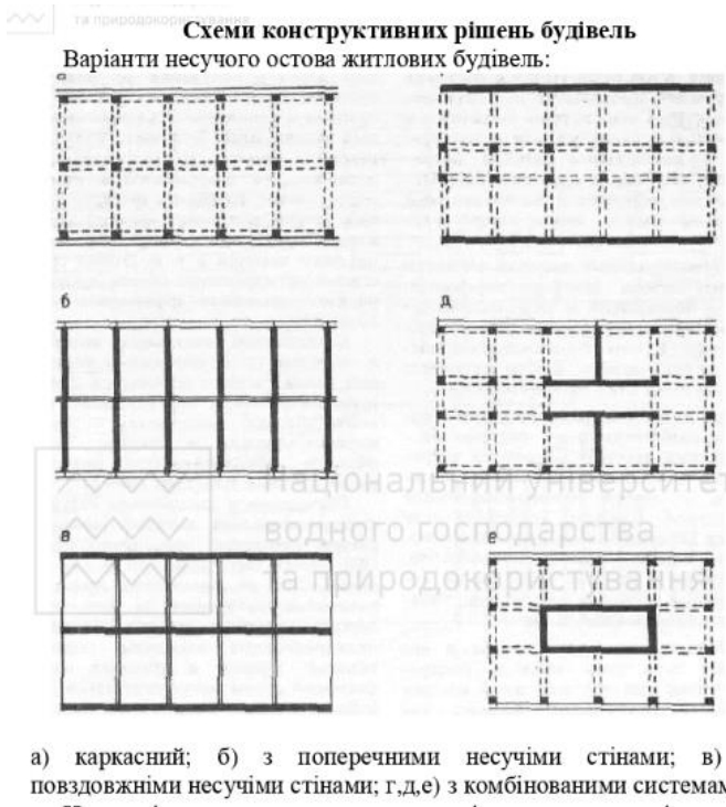
Рис. 6. Схеми конструктивних рішень будівель
