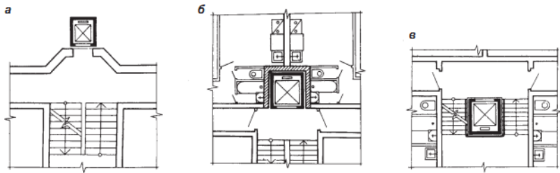
Рис. 21. Схеми розміщення ліфтових шахт: а, б - у торці сходової клітини, в - в середині сходової клітини
