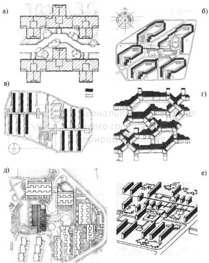
Рис. 13. Приклади блокування секцій при різній забудові території
