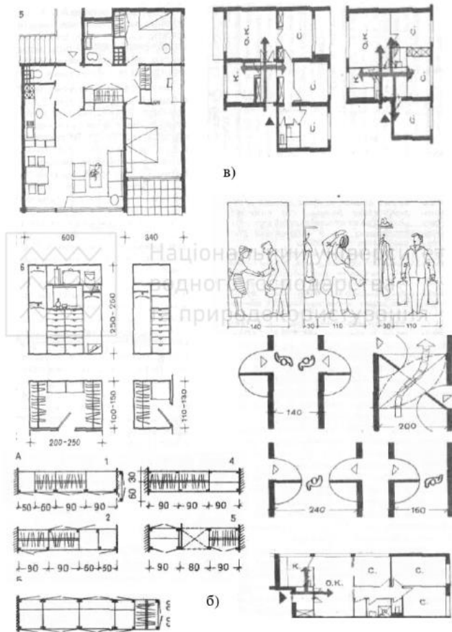
Рис. 9. Приклади: а - квартира із вбудованими шафами, б - габарити гардеробних кімнат, в - визначення габаритів прихожої
