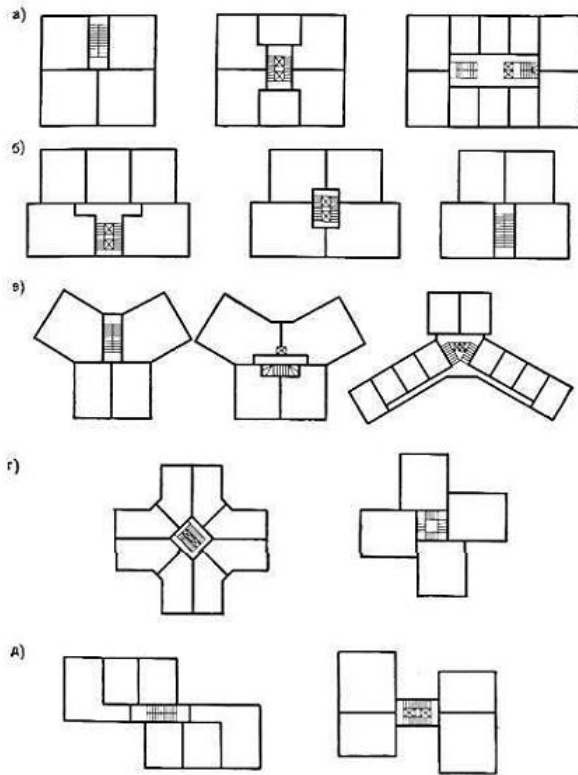
Рис. 5. Форми планів одnoseкційних будинків: а - прямокутні, б - Т-подібні, в - променеподібні, г - хрестоподібні, д - пароблочні
