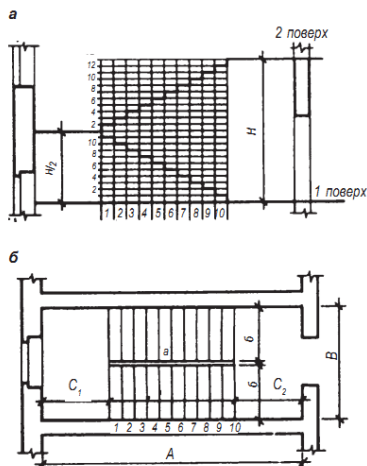
Рис. 10.4. Схема розбивки сходів: а – в розрізі; б – у плані
