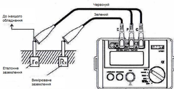
Рисунок 6 – Підключення приладу по двопровідній схемі
