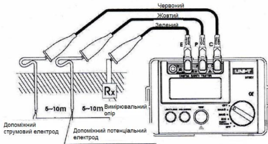
Рисунок 5 – Підключення приладу по трьох провідній схемі
