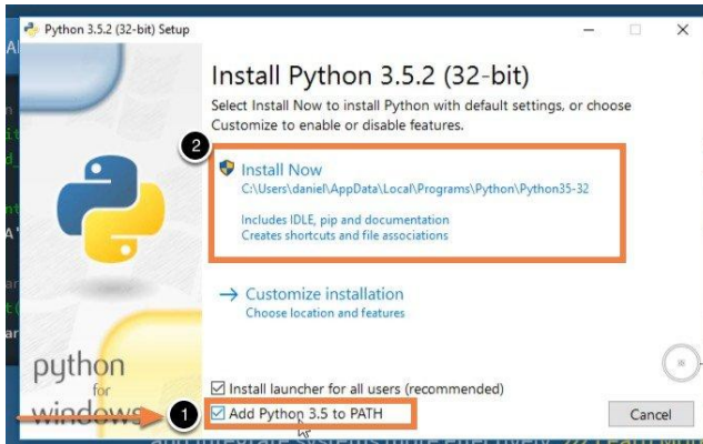
Рис. 1.1. Інсталяція Python
