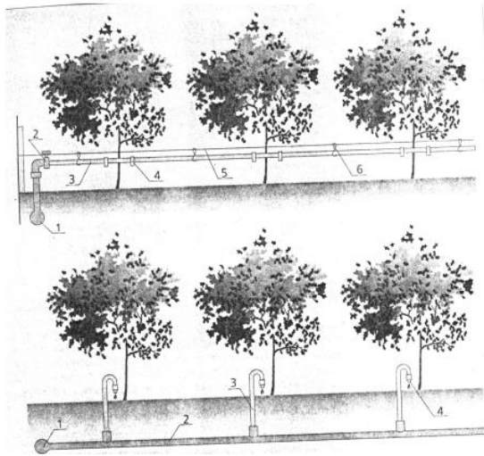
Рис. 99 Схеми розміщення поливних трубопроводів системи крапельного зрошення:
