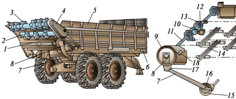
Рис. 1. Кузовний розкидач ПРТ-10:
