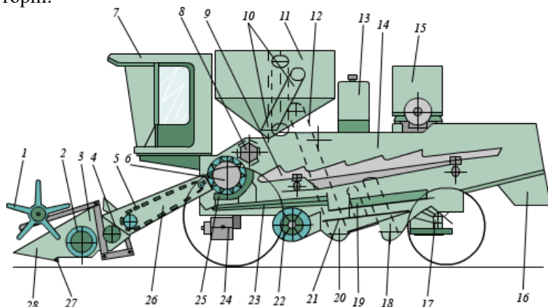
Рис. 2. Функціональна схема зернозбирального комбайна КЗС-9-1: 1 - мотовило; 2 - шнек; 3 - корпус жниварки; 4 - бітер приставки; 5 - транспортер похилої камери; 6 - молотильний барабан; 7 - кабіна; 8 - відбійний бітер; 9 - соломотряс; 10 - вивантажувальний шнек; 11 - бункер; 12 - зерновий елеватор; 13 - паливний бак; 14 - камера соломотряса; 15 - двигун; 16 - капот; 17 - міст напрямних коліс; 18 - колосовий шнек; 19 - домолочувальний пристрій; 20 - зерновий шнек; 21 - решета очищення; 22 - вентилятор; 23 - струшувальна дошка; 24 - міст
