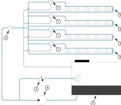
Рис. 13. Безпервна циркуляція в гідравлічній системі (СН):
