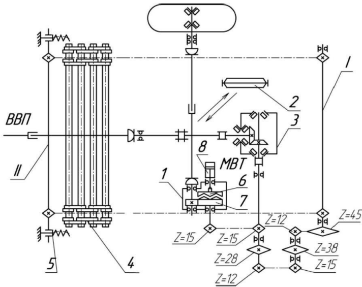
Рис. 7. Кінематична схема механізму приводу транспортера:
