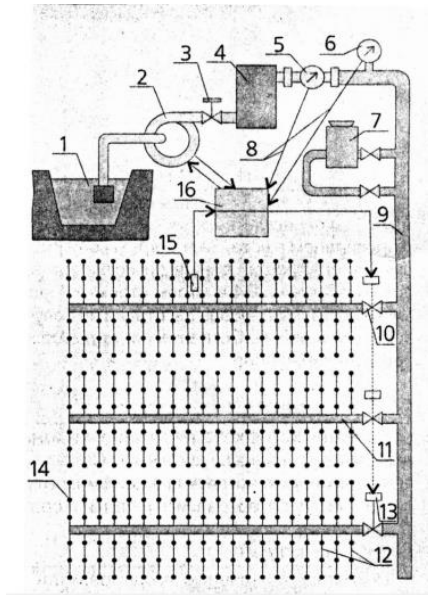
Рис. 1 Принципова схема системи крапельного зрошення: 1-водозабірний вузол; 2-насос; 3-засувка; 4-фільтр; 5-лічильник витрачання води; 6-манометр; 7-пристрій для приготування та подачі добрив у трубопровідну мережу; 8-канали зв'язку; 9-магістральний трубопровід; 10-дистанційно керована засувка; 11- розподільчий трубопровід; 12-поливний трубопровід; 13-блок керування засувкою; 14-крапельниця; 15-датчик необхідності поливу; 16-пульт управління.
