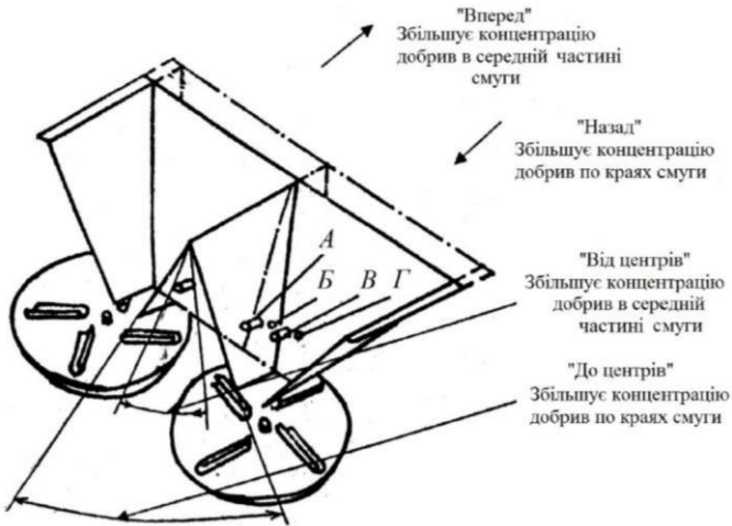
Рис. 6. Схема регулювання туконапрямника.
