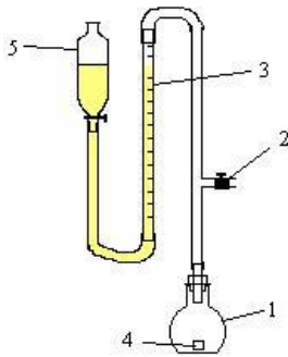
Рис. 7.2. Газометрична установка для визначення активності каталази
