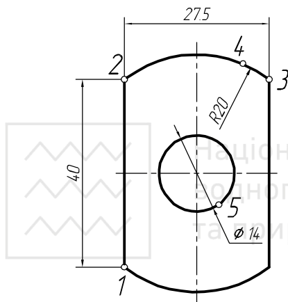
Рис. 1.30. Нанесення розмірів
