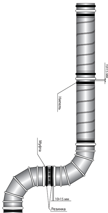
Рис. 35. Монтаж системи повітропроводів з гумовим ущільнювачем
