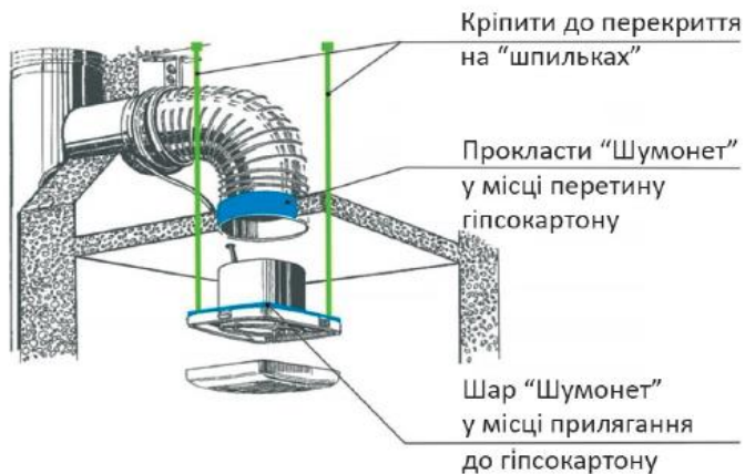
Рис. 40. Схема приєднання вентилятора до жорсткого повітропроводу
