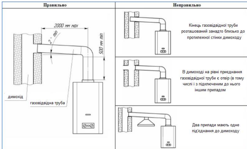
Рис. 44. Приєднання газового нагрівача води до димоходу
