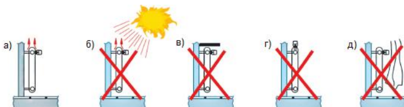
Рис. 12. Вимоги до розташування радіаторів із стандартними терморегуляторами
