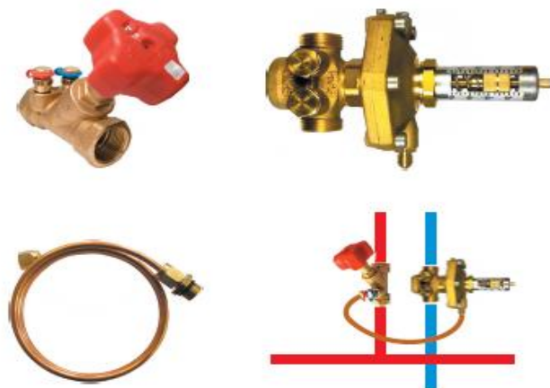
Рис. 24. Встановлення автоматичного регулятора перепаду тиску
