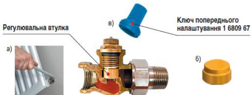
Рис. 6. До монтажу термостатичних клапанів
