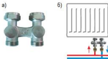
Рис. 20. Радіаторний клапан HERZ-3000-RL-1
