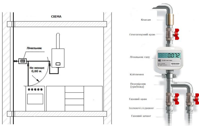
Рис.46. Варіанти встановлення лічильника газу [25]
