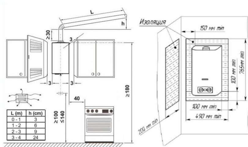
Рис.43. Встановлення газового нагрівача води
