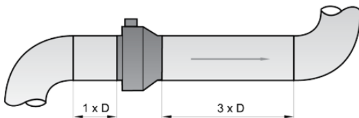
Рис. 34. Мінімальні рекомендовані довжини прямих ділянок повітропроводу до і після вентилятора
