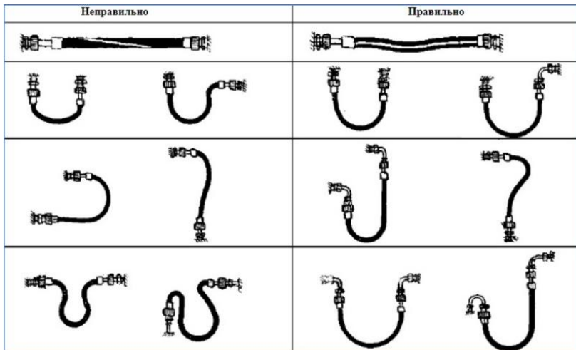
Рис. 45. Приєднання гнучких підведень до газового нагрівача води
