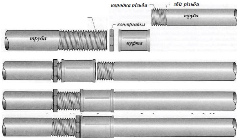
Рис. 41. З'єднання сталевих труб за допомогою згону
