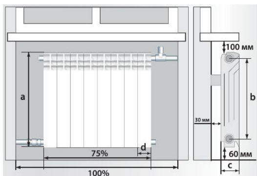
Рис. 27. Вимоги щодо розташування опалювальних приладів
