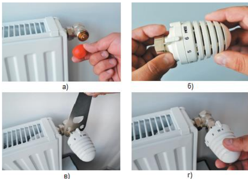
Рис. 14. Монтаж стандартної термоголовки із вбудованим датчиком температури
