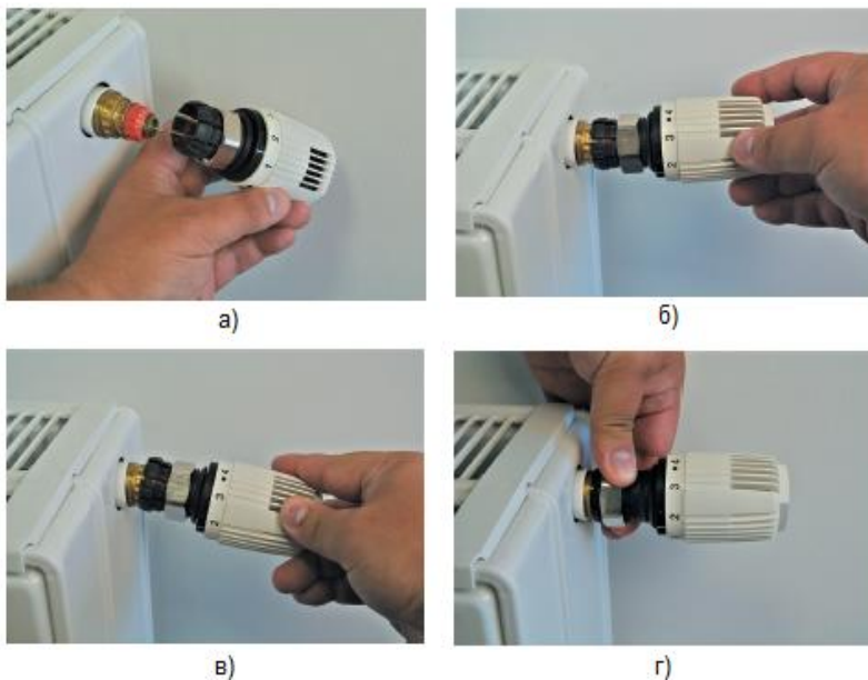
Рис. 15. Монтаж термоголовок HERZ “D” на буксу Danfoss RA-N
