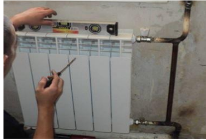
Рис. 31. Перевірка встановлення опалювального приладу за рівнем
