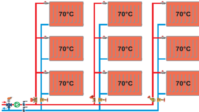
Рис. 22. Збалансована статична система опалення
