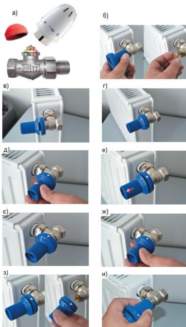
Рис. 7. Гідравлічне налаштування термостатичного клапана
