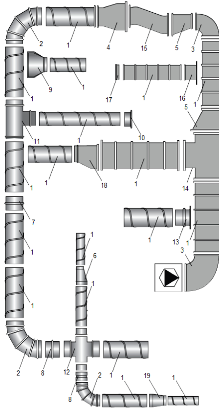
Рис. 38. Монтажна схема системи повітропроводів:
