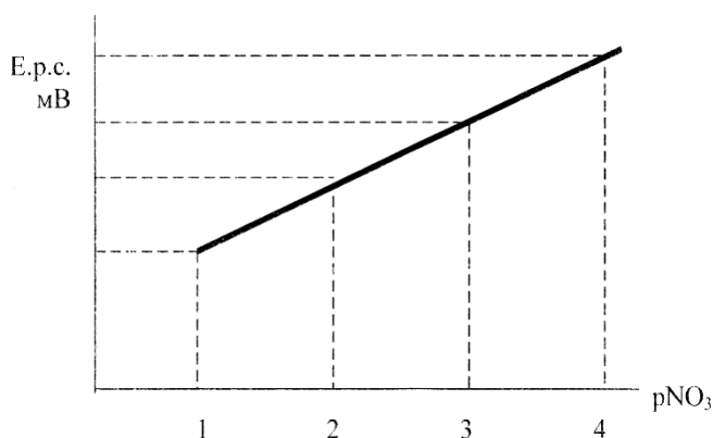
Рис.1. Калібувальний графік
