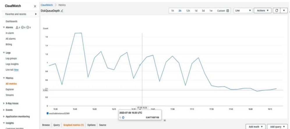
Рис. 2. Метрика DiskQueueDepth
