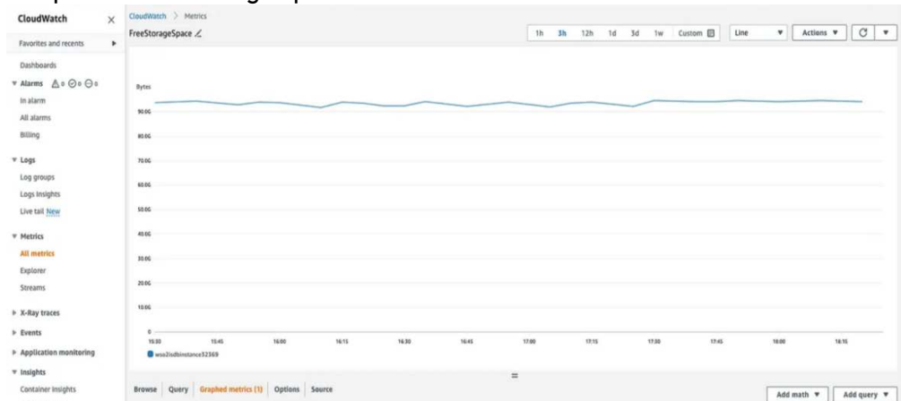
Рис. 4. Метрика FreeStorageSpace
