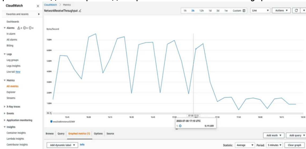
Рис. 5. Метрика NetworkReceiveThroughput
