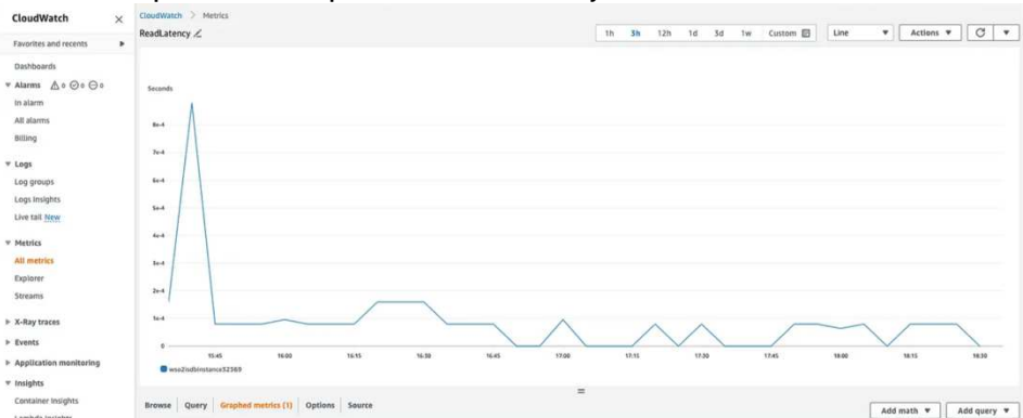
Рис. 6. Метрика ReadLatency
