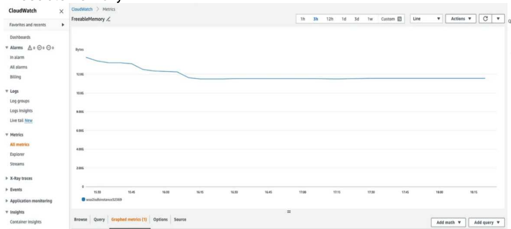
Рис. 3. Метрика FreeableMemory
