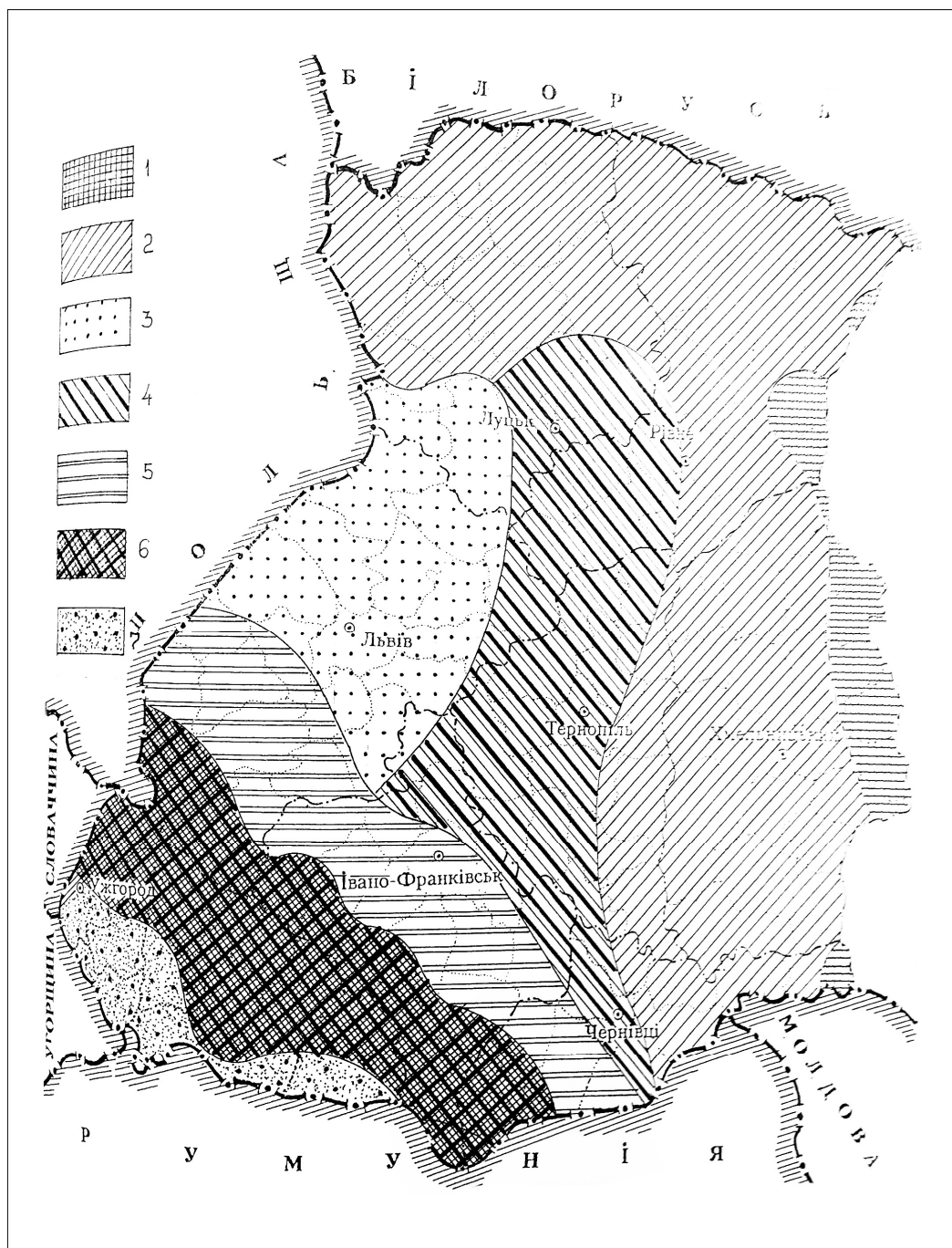
Рис. 5.1. Геологія регіону
