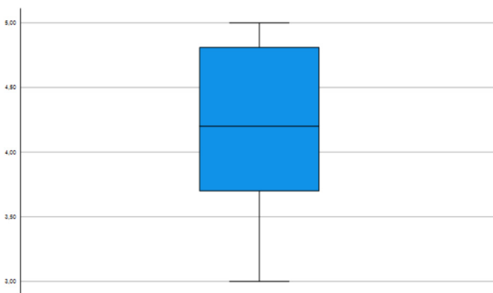
Fig. 2. Boxplot
