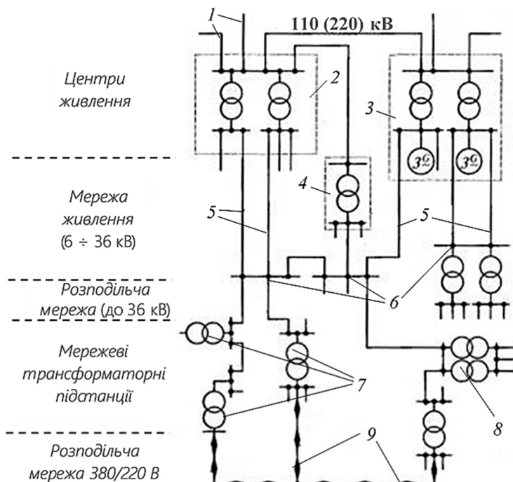
Рис. 6.4. Принципова схема електропостачання міста:
