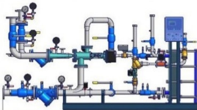
Рис. 5.8. Гідроелеваторний тепловий вузол з автоматичним регулюванням температури і витрат теплоносія
