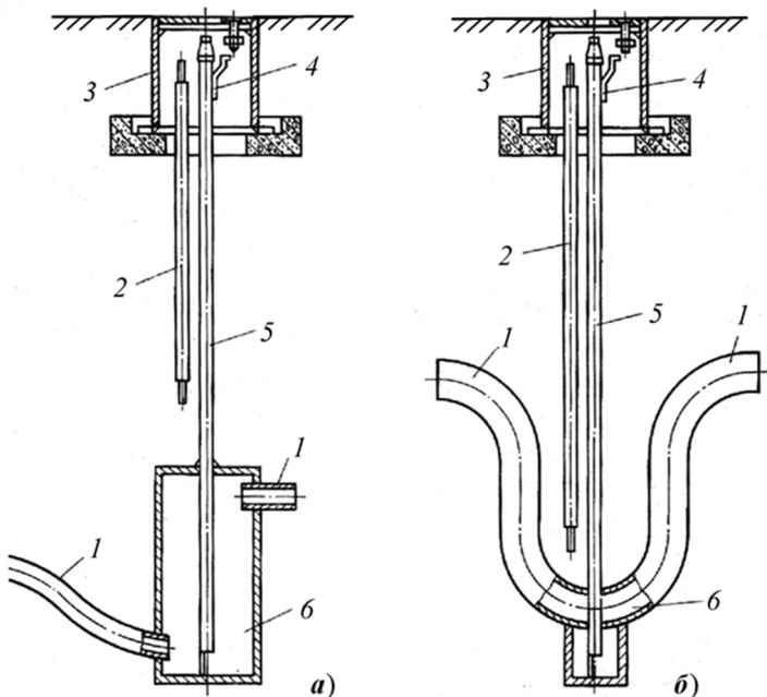
Рис. 4.8. Гідрозатвори:
