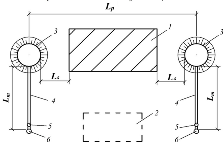
Рис. 2.22. Розташування пожежних резервуарів біля будівель:
