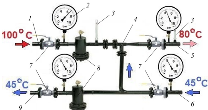
Рис. 5.7. Гідроелеваторний тепловий вузол:
