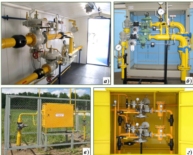
Рис. 4.4. Пункти регулювання газу (ПРГ):
