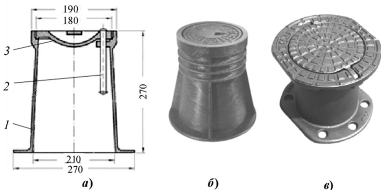
Рис. 4.7. Ковери газові:
