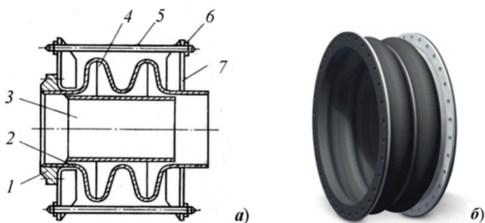
Рис. 4.9. Лінзовий ( а ) та гумокордовий ( б ) компенсатори:
