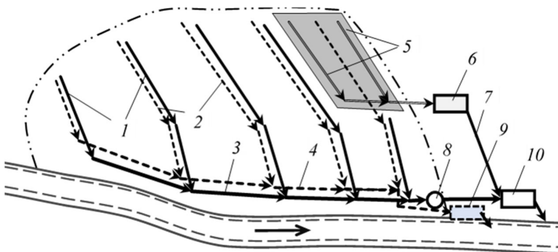
Рис. 3.4. Схема повної роздільної системи водовідведення
