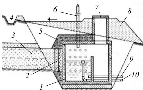
Рис. 2.6. Низхідний каптаж:
