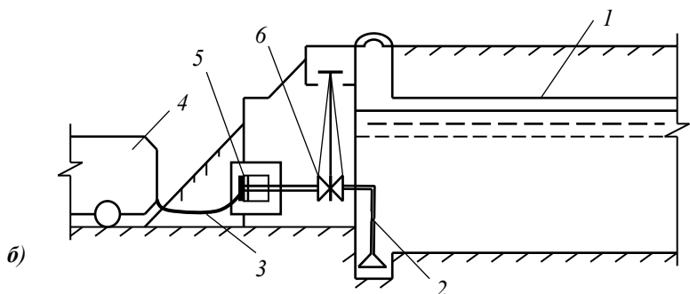
Рис. 2.21. Загальний вигляд (а) наземних пожежних резервуарів та схема відбору води із них (б):
