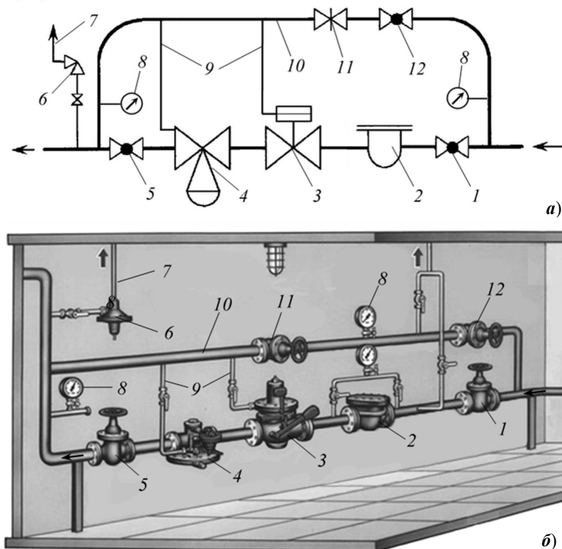
Рис. 4.5. ГРП і ГРУ: а) принципова схема; б) загальний вигляд технологічного обладнання;
