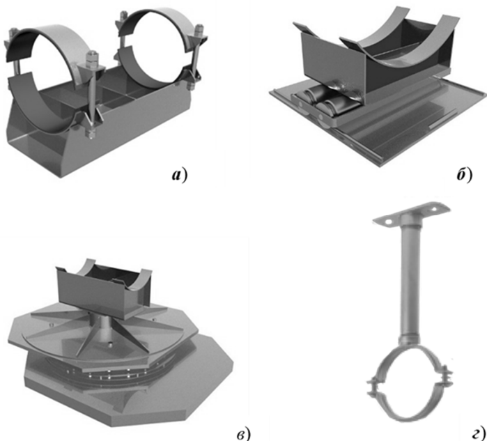
Рис. 5.12. Рухомі опори теплових мереж: а) ковзна; б) коткова; в) кульова; з) підвіска
