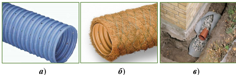
Рис. 3.13. Пластмасові дренажні труби: а) з дірчатою перфорацією; б) із захисним волокнистим кожухом; в) з дренажною обсыпкою і геотекстилем
