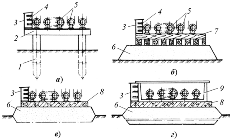
Рис. 5.6. Надземне прокладання інженерних мереж:
