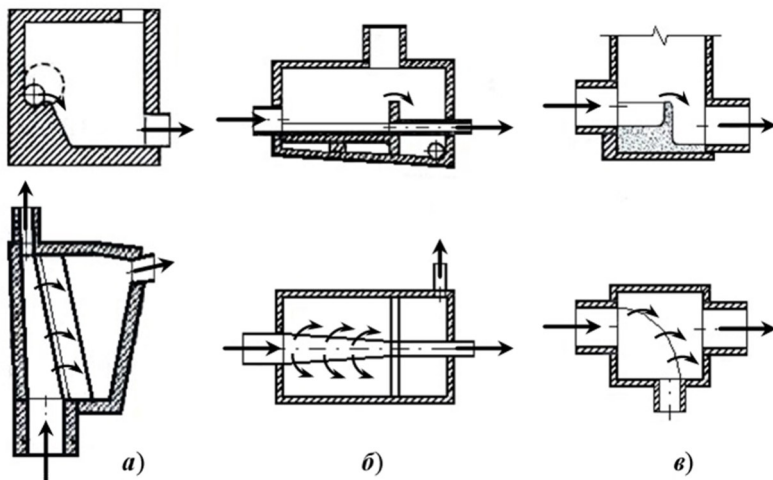
Рис. 3.6. Типи розподільчих камер з водозливами:
