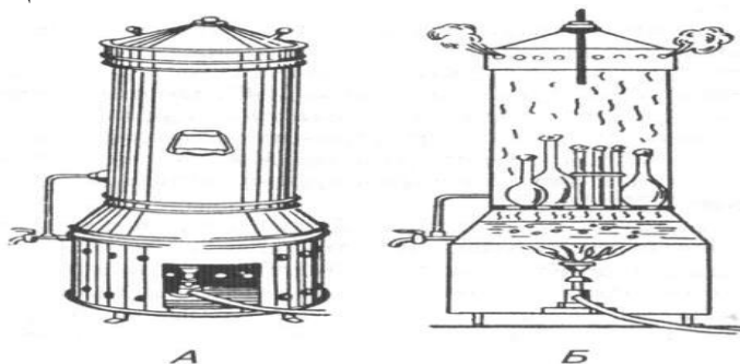
Рис. 1 Апарат Коха: А - зовнішній вигляд; Б - внутрішня будова
