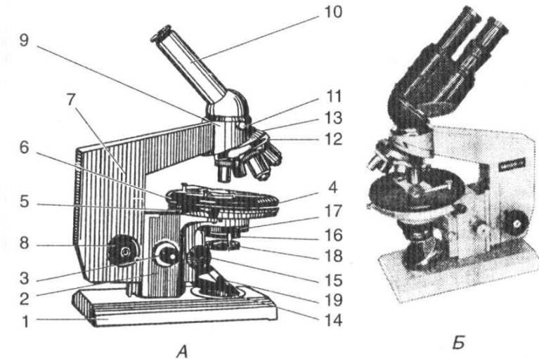
Рисунок 3 Біологічні мікроскопи серії «БИОЛАМ» (А - МБР-1; Б- МБР-3): 1 - основа; 2 - коробка з механізмом мікрометричного фокусування; 3 - рукоятка мікрогвинта; 4 -
