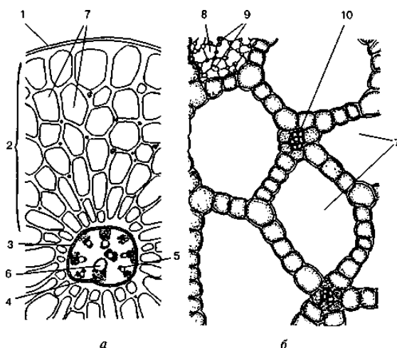
Рис. 5. Будова стебла рдесника:
