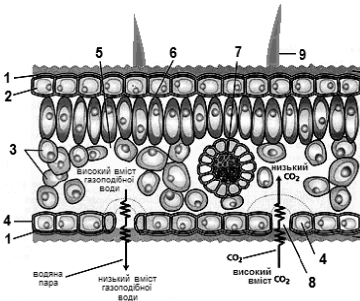
Рис. 4. Будова пластинки листка
