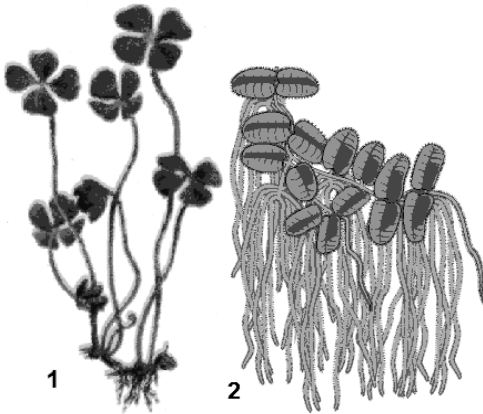
Рис. 3. Водні папороті: 1 – марсилія чотирилиста ( Marsilea quadrifolia ), 2 – сальвінія плаваюча ( Salvinia natans )
