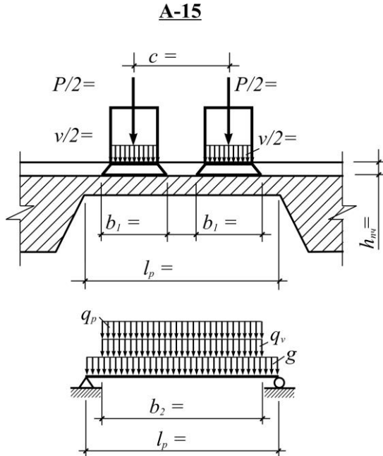
Рис.6. Схема розрахунку плити на тимчасове рухоме навантаження А-15
