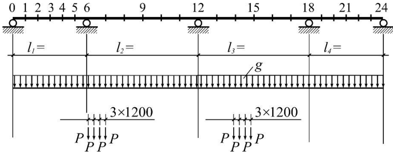
Рис. 15. Схема навантаження при визначенні поперечної сили від НК
