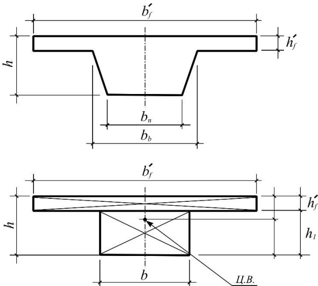
Рис. 9. Схема приведення реального перерізу до приведенного
