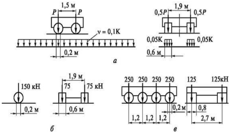
Рис. Схеми тимчасових навантажень для розрахунку автодорожніх і міських мостів: а – автомобільне навантаження АК; б – одинична вісь для перевірки елементів проїзної частини; в – НК-100
