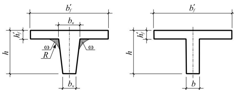
Рис.8 . Схема до визначення розмірів приведенного перерізу
