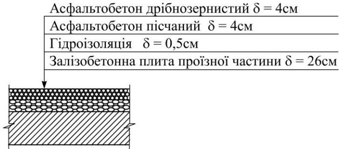
Рис.4. Конструкція дорожнього одягу
