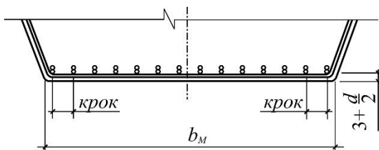
Рис. 16. Схема розташування арматури для нижнього поясу балки
