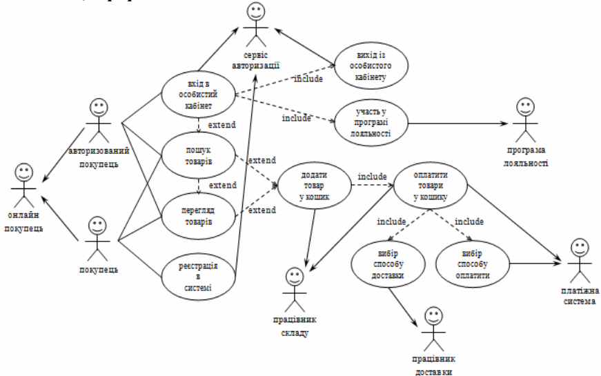
Рис. 2.2. Діаграма варіантів використання «купівля товарів»
