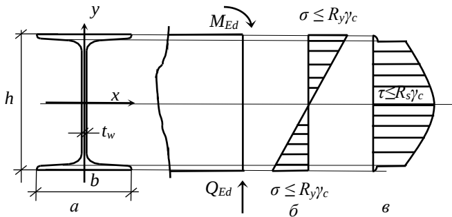
Рис. 2. Напружено-деформований стан балки 1-го класу: a – форма суцільного поперечного перерізу; \bar{\sigma} – епюра \sigma ; \bar{\tau} – епюра \tau
