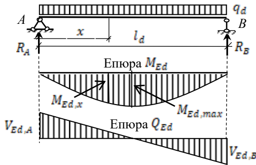
Рис. 1. Епюра моментів та поперечних сил в однопролітній балці
