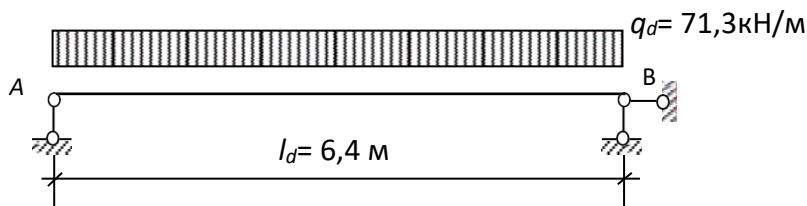
Рис. 8. Розрахункова схема балки
