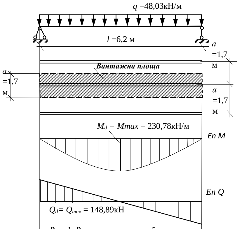
Рис. 1. Розрахункова схема балки
