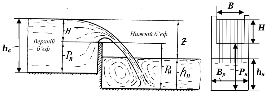
Рис. 1. Схема водозливу
