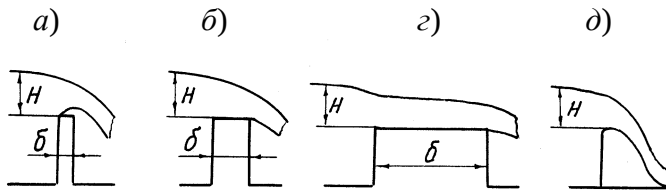
Рис. 2. Схеми водозливів
