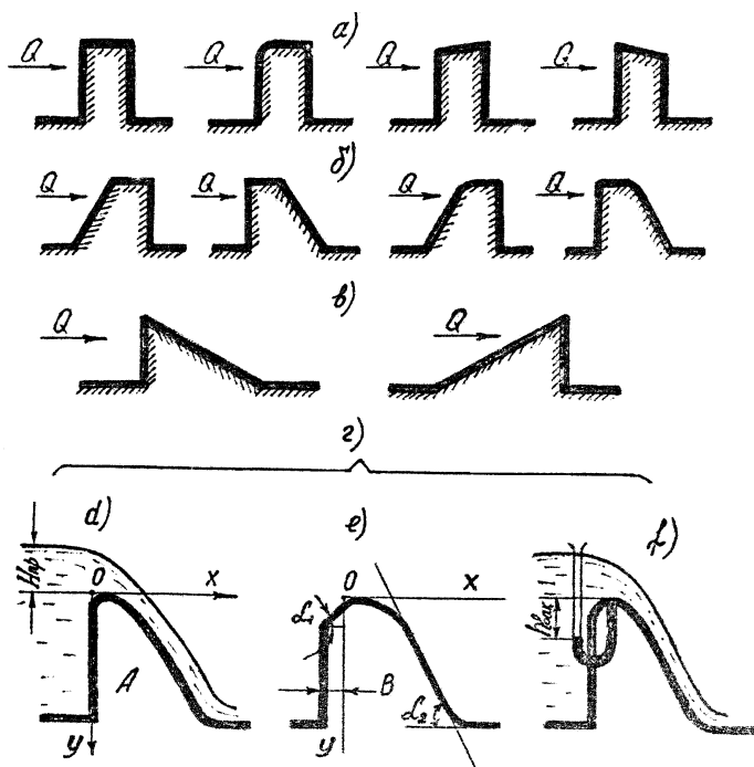
Рис. 5. Водозливи практичного профілю
