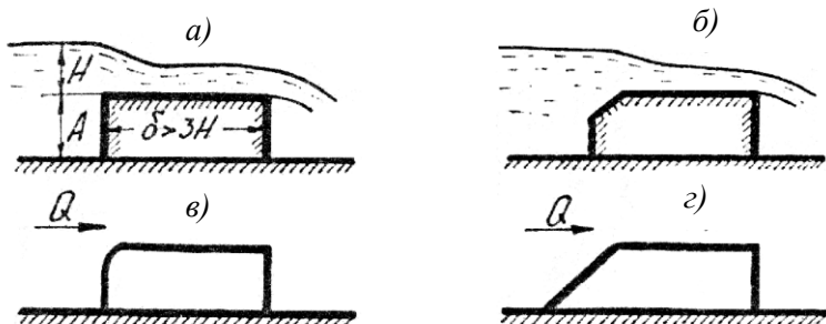
Рис. 7. Типи водозливів з широким порогом
