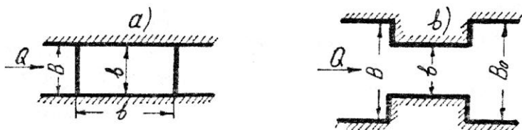
Рис. 8. Водозливи з широким порогом без бокового стиснення (а) та з боковим стисненням (b)
