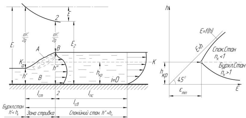
Рис. 5. Схема досконалого гідралічного стрибка та його внутрішня структура
