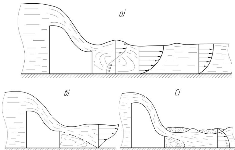
Рис. 9. Схеми розподілу швидкостей руху рідини для різних режимів спряження б'єфів а/
