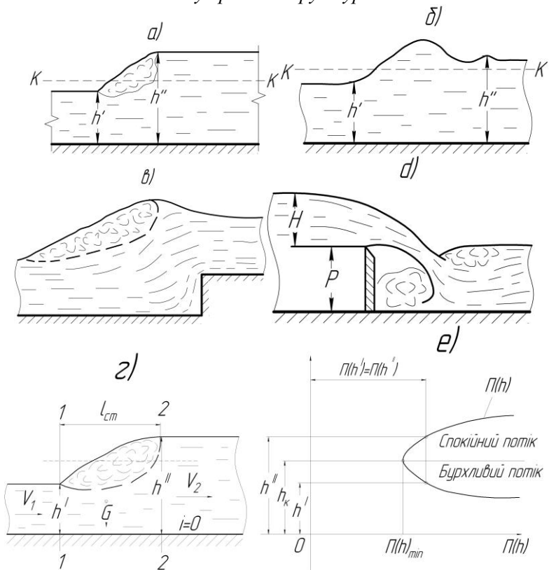
Рис. 6. Схеми видів гідралічного стрибка та графік функції гідралічного стрибка
