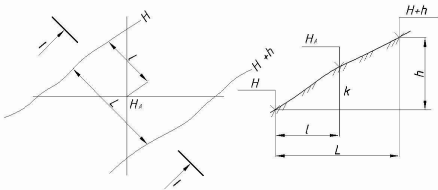
Рис.5.1. Визначення відміток поверхні землі H_A вершин квадратів методом інтерполяції.
