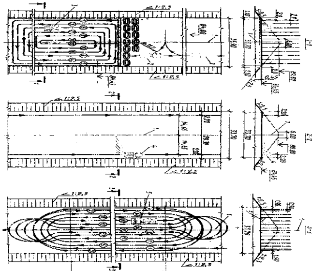
Рис. 5.10.Схема пошарового ущільнення ґрунту греблі:
