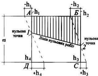
Рис.5.3 Графічне визначення точок нульових робіт
