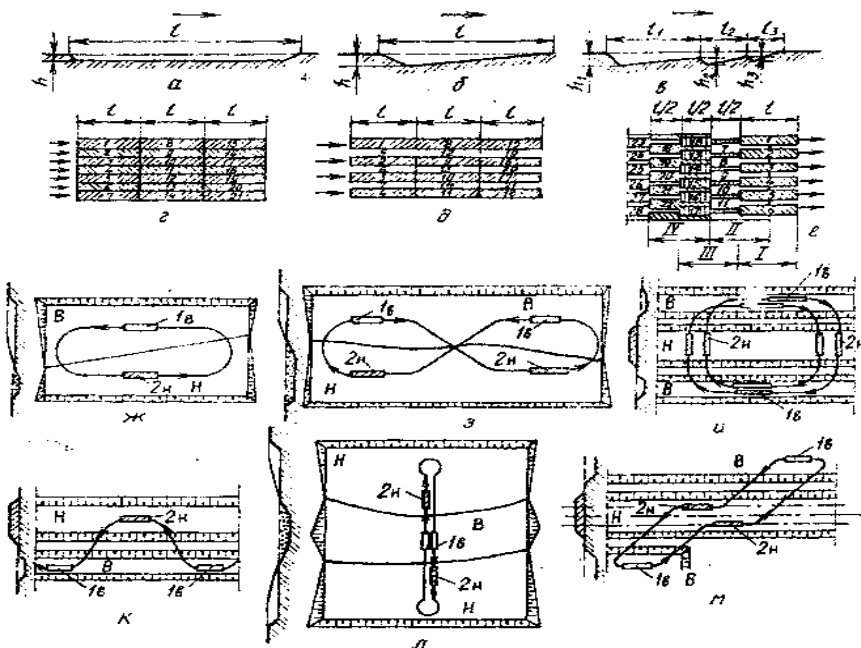
Рис. 5.6. Способи різання ґрунту скрепером і схеми руху а - різання тонкою стружкою постійної товщини; б - теж, клиновидним профілем; в - теж, гребінчастим профілем; г - проходки поздовжні, д - теж, через полосу, е - теж, ребристо-шахматні; ж - рух по еліпсу, з - теж, по вісімці; и - теж, по спіралі, к - теж, по зигзагу, л - теж, поперечно - човниковий; м - теж, повздожньо - човниковий, L - довжина шляху завантаження ковша; I..IV- ряди проходок скрепера, 1..28 - послідовність набирання ґрунту, Н - насип; В - виїмка; 1в - набирання ґрунту; 2н - розвантаження (відсипання) ґрунту, h, \dots, h_3 - товщина стружки.
