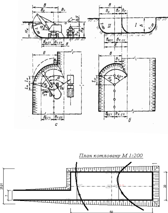
Рис. 5.8. Схема бокових экскаваторних забоїв екскаватора пряма лопата при розробці котлованів:
