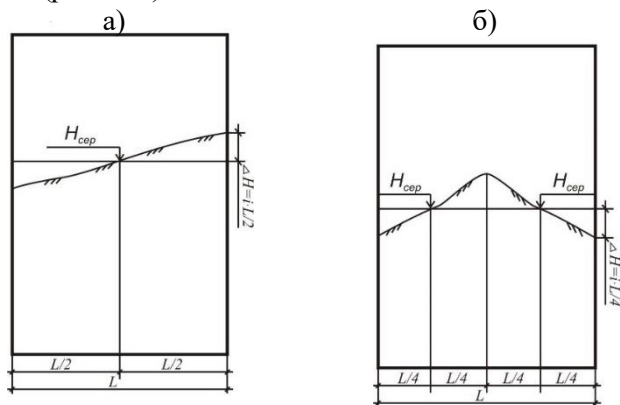
Рис.5.2. Визначення проектних (червоних) позначок:
