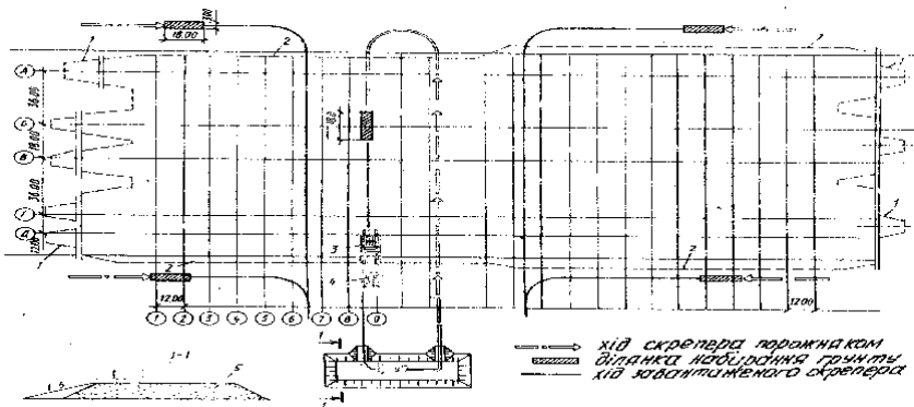
Рис.5.5. Схема зрізання родючого шару:
