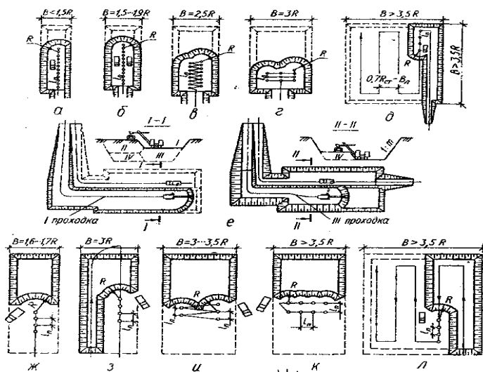
Рис. 5.7. Розробка котлованів одноковшовими екскаваторами:
