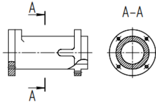
Рис.3.5. Положення січної площини розрізу Зображення розрізу та перерізу
