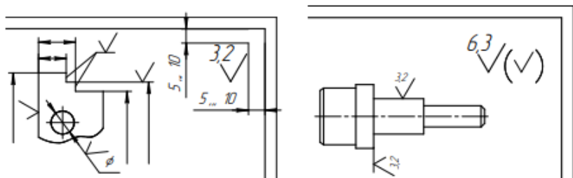
Рисунок 3.7 – Позначення шорсткості
