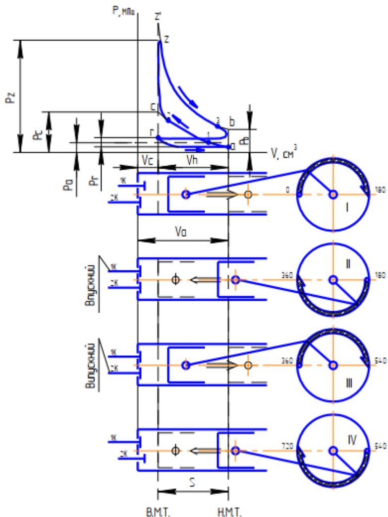
Рис.6.2. Індикаторна діаграма і схема роботи бензинового двигуна: I – впуск; II – стиснення; III – розширення; IV – випуск.
