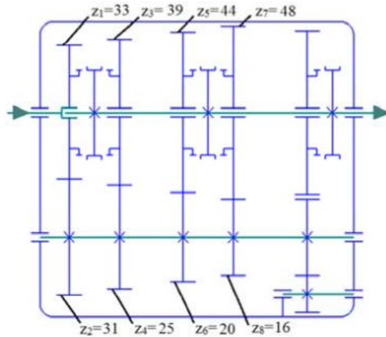
Рис. 5.1. Приклад виконання кінематичної схеми базової КП проектного ТЗ
