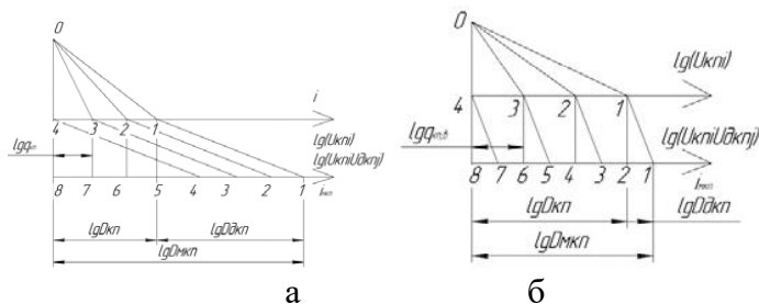
Рис. 5.2. Лінійні діаграми для проектованої КМ: а - задня додаткова КП; б - передня додаткова КП
