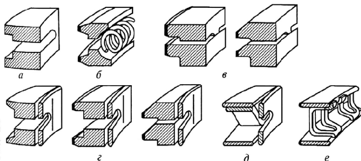
Рис. 1.9. Конструктивне виконання маслоснімних кілець :
