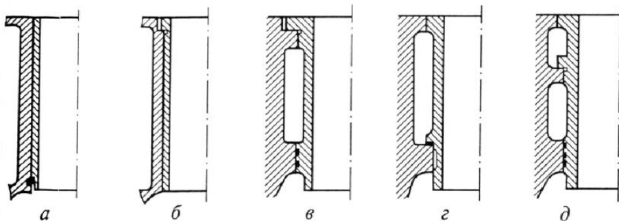
Рисунок 1.2. Типи гільз циліндрів:
