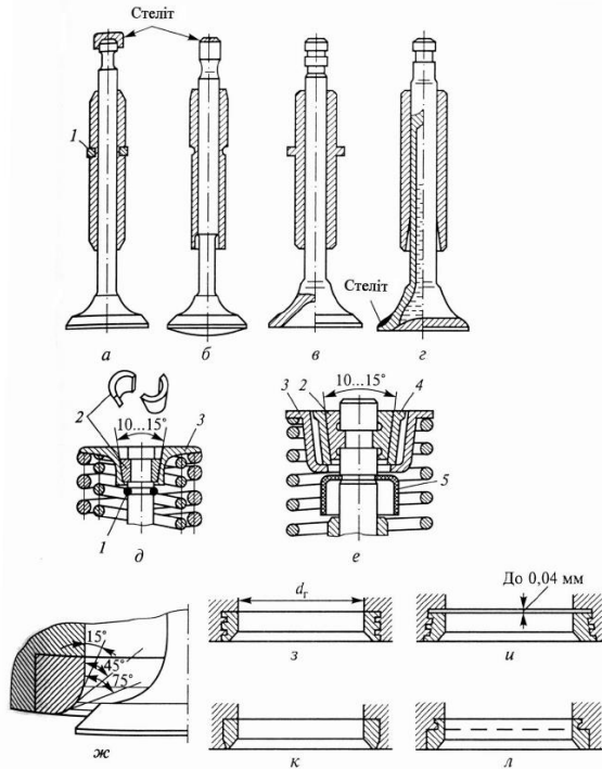
Рис. 2.4. Елементи клапанного механізму: а-г – клапани, д-е – деталі кріплення тарілки пружини клапана; ж-л – сидла клапанів; 1 – пружинне стопорне кільце; 2 – сухарі; 3 – опорна тарілка; 4 – втулка; 5 – маслознімний ковпачок
