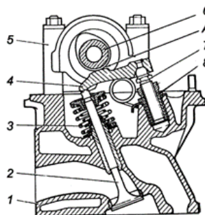
Рис. 2.3. ГРМ з верхнім розташуванням розподільних валів: 1 – головка циліндрів; 2 – клапан; 3 – ущільнюючий ковпачок; 4 – одноплечий важіль клапана (рокер); 5 – корпус опор розподільного валу; 6 – розподільний вал; 7 – регулювальний гвинт; 8 – контргайка; А – тепловий зазор між важелем і кулачком розподільного валу
