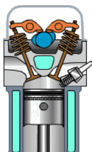
Рис. 2.3. ГРМ з верхнім розташуванням розподільних валів: 1 – головка циліндрів; 2 – клапан; 3 – ущільнюючий ковпачок; 4 – одноплечий важіль клапана (рокер); 5 – корпус опор розподільного валу; 6 – розподільний вал; 7 – регулювальний гвинт; 8 – контргайка; А – тепловий зазор між важелем і кулачком розподільного валу
