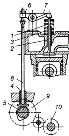
Рис. 2.2. ГРМ з верхнім розташуванням клапанів: 1 – клапан; 2 – напрямна втулка; 3 – пружина; 4 – штовхач; 5 – кулачок розподільного валу; 6 – регулювальний гвинт; 7 – натискний важіль (коромисло); 8 – штанга; 9 – шестерня розподільного валу; 10 – шестерня колінчастого валу
