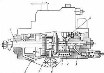
Рис. 4.4. Розподільний насос з аксіальним рухом плунжера: 1 – вал приводу; 2 – важіль регулятора; 3 – плунжер; 4 – дозатор; 5 – пружина; 6 – кулачкова шайба; 7 – ролик; 8 – шиберний паливopідкачувальний насос
