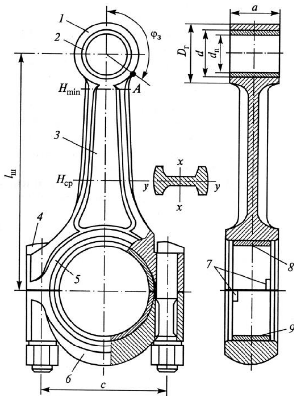
Рис. 1.11. Конструкція шатуна:
