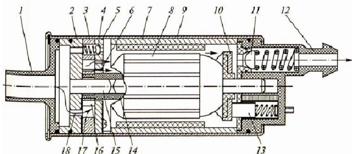
Рис. 3.4. Електричний паливний насос: 1 – підвідний штуцер; 2 – основа; 3 – статор насоса; 4 – запобіжний клапан; 5 – кришка; 6 – вихідний канал; 7 – статор електродвигуна; 8 – якір електродвигуна; 9 – корпус; 10 – колектор; 11 – зворотний клапан; 12 – напірний штуцер; 13 – щітка; 14 – муфта; 15 – вал; 16 – сепаратор; 17 – ролик; 18 – вхідний канал
