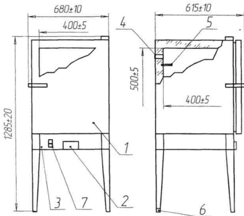
Рис. 1.1 - Шкаф сухоповітряна ШС-80-КЗМА: 1 – корпус; 2 – пульт (індикатор температури); 3 – підсвітка; 4 – отвір для відведення пару; 5 – датчик температури; 6 – опорний гвинт; 7 – вимикач.
