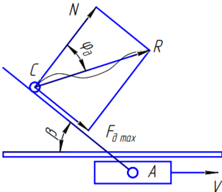
Рис.3.5 - До визначення динамічного кута тертя
