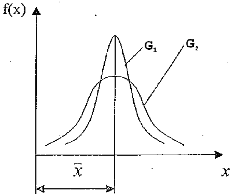
Рис. 5.1 – Криві нормального розподілу випадкової величини
