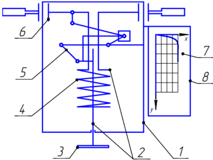
Рис. 2.2 - Схема твердоміра Ю.Ю. Ревякіна : 1 – напрямна штанга; 2 – телескопічна штанга; 3 – наконечник; 4 – пружина; 5 – записувальні ланки; 6 – тримачі; 7 – лист міліметрівки; 8 – планка
