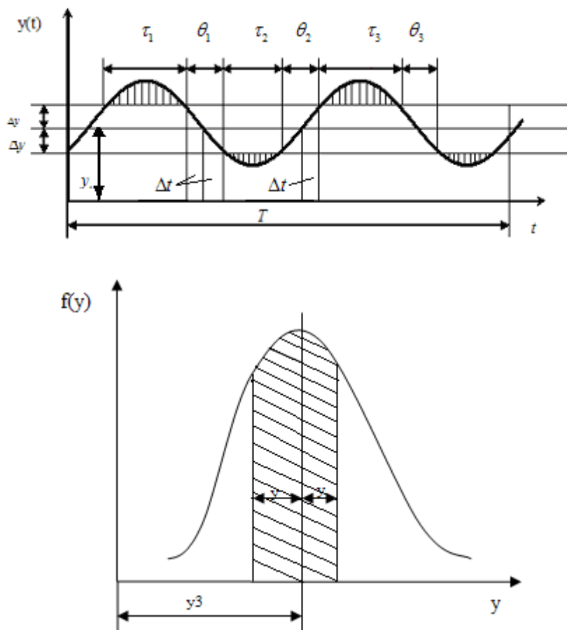
Рисунок 6.1 - Реалізація якості роботи y(t) сільськогосподарської машини (а) і одновірною щільністю цієї реалізації (б)
