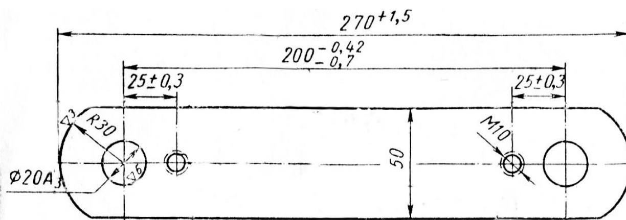
Рисунок 7 – Зовнішня пластина
