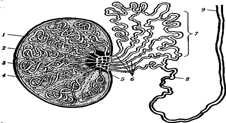
Мал. 36. Схема будови сім'яника:
