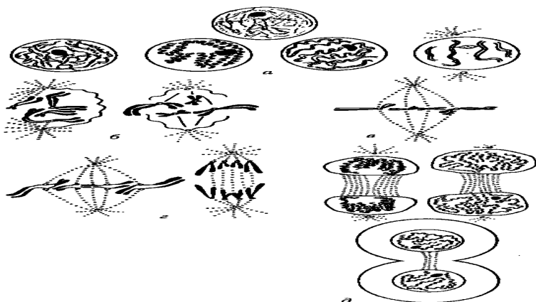
Рис. 1. Схема мітотичних фаз у тваринній клітині: а — профаза; б — прометафаза; в — метафаза; г — анафаза; д — телофаза.
