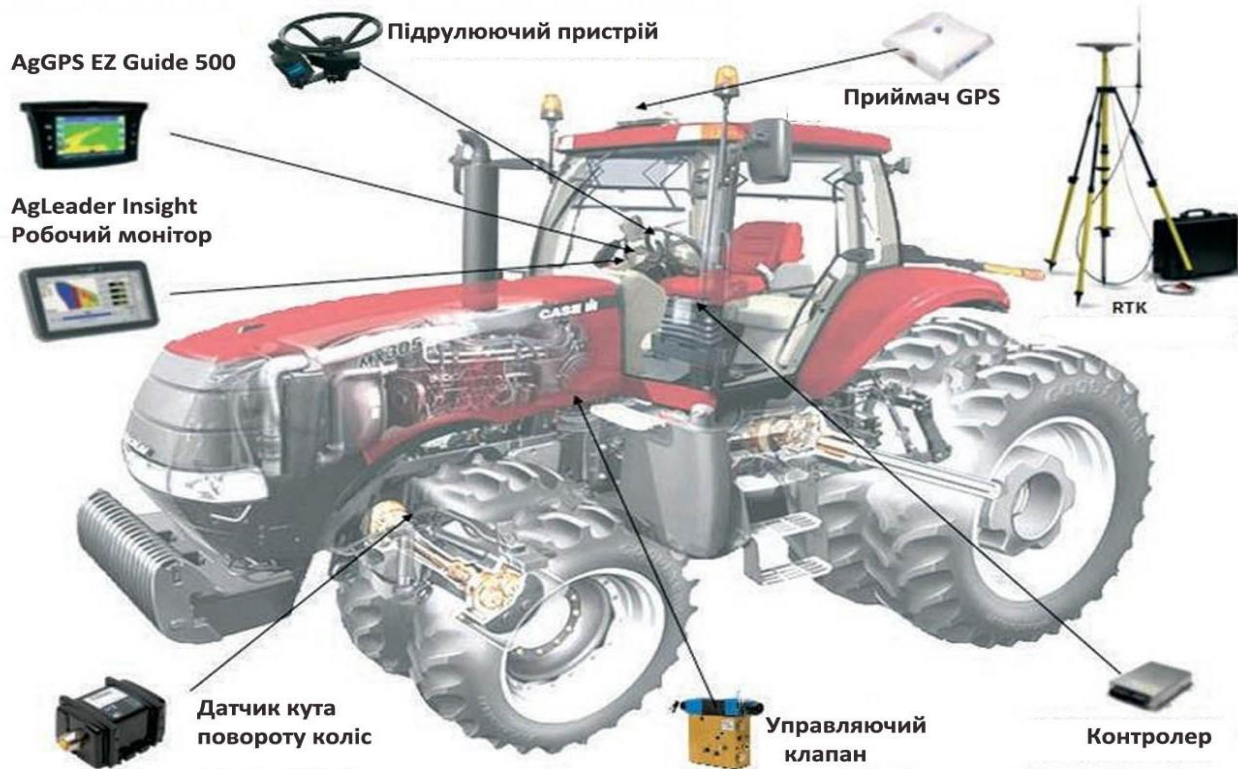
Рис. 21 Загальна компоновка автопілота на прикладі Case Магнит з диференціальною корекцією RTK
