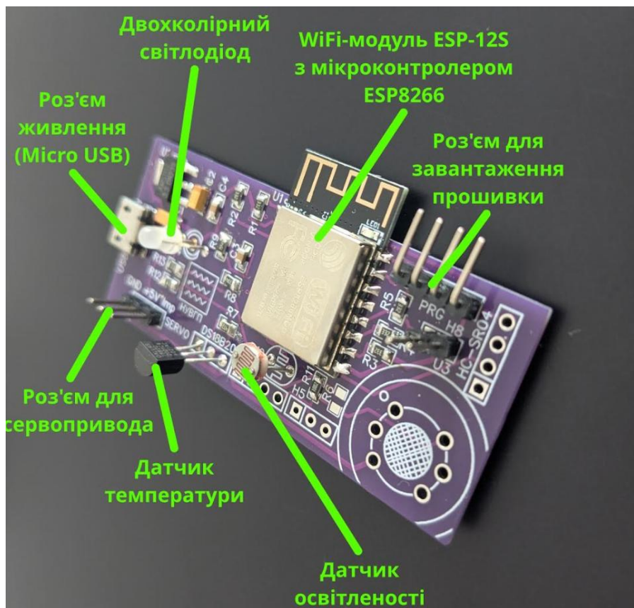
Рис.13.1. Мікропроцесорна плата з мікроконтролером ESP8266 та датчиками температури й освітленості
