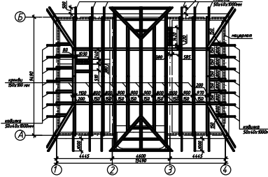
План крокв М1:100
