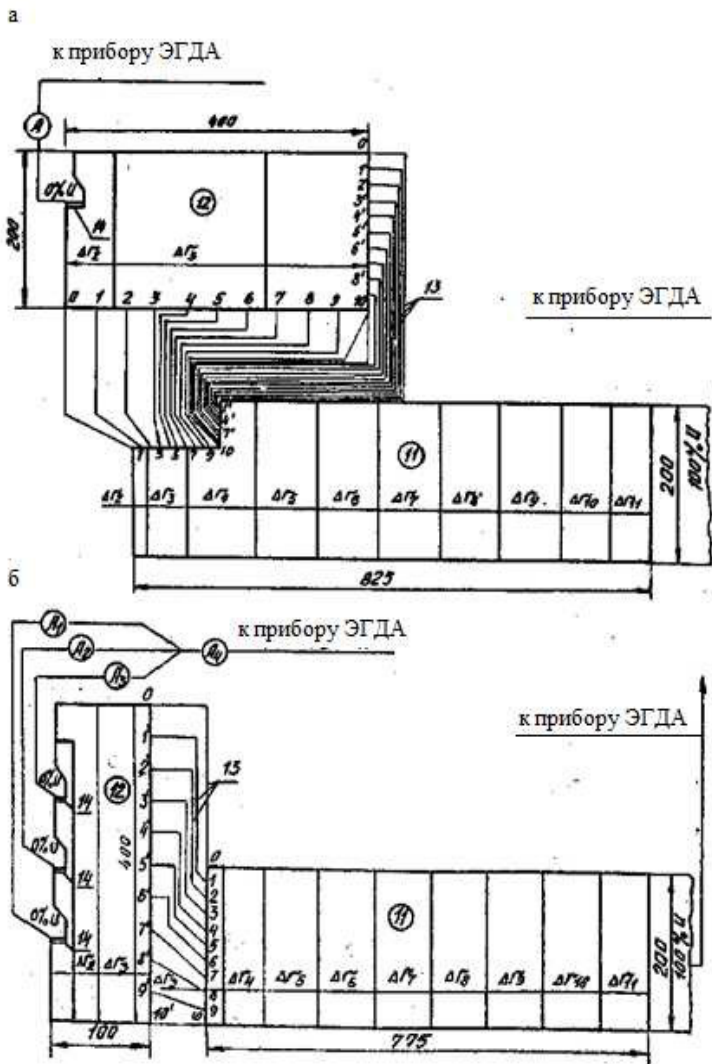
Рис. 6. Модели ЭГДА для исследования скважины с ФУГЗ: 0...10 – контактные соединения; 11 – пласт; 12 – прискважная зона; 13 – провода; 14 – шина Панчишина; А – миллиамперметры
