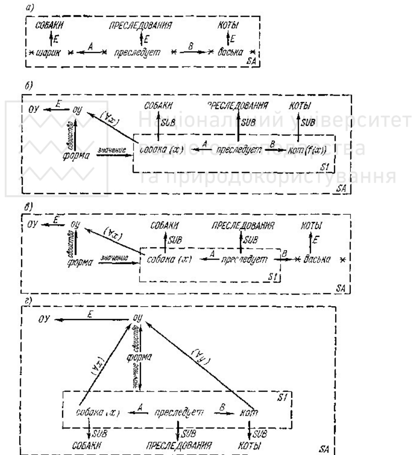
Рис. 10.24. К разбиению семантической сети на пространство.
