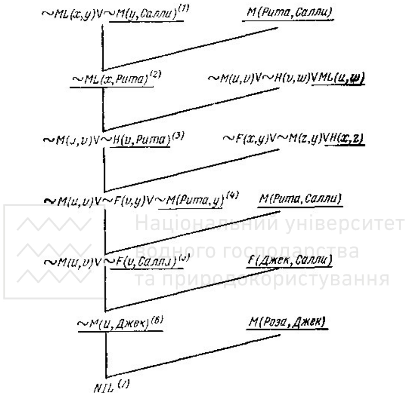
Рис. 12.8 Использование констант для ведения поиска.
