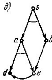
Рис. 11.3. Пример работы алгоритма: а) исходный граф, б), в), г) шаги алгоритма, д) решающий граф.
