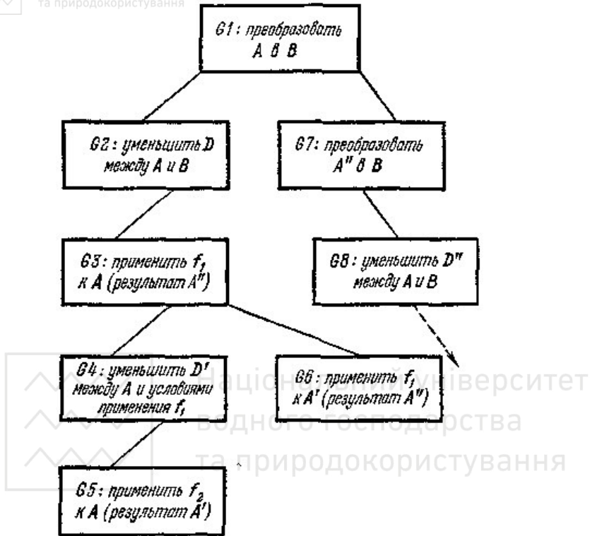
Рис. 10.7. Пример работы механизма редукции.
