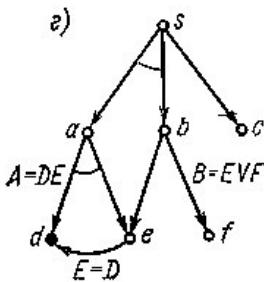
Рис. 11.3. Пример работы алгоритма: а) исходный граф, б), в), г) шаги алгоритма, д) решающий граф.
