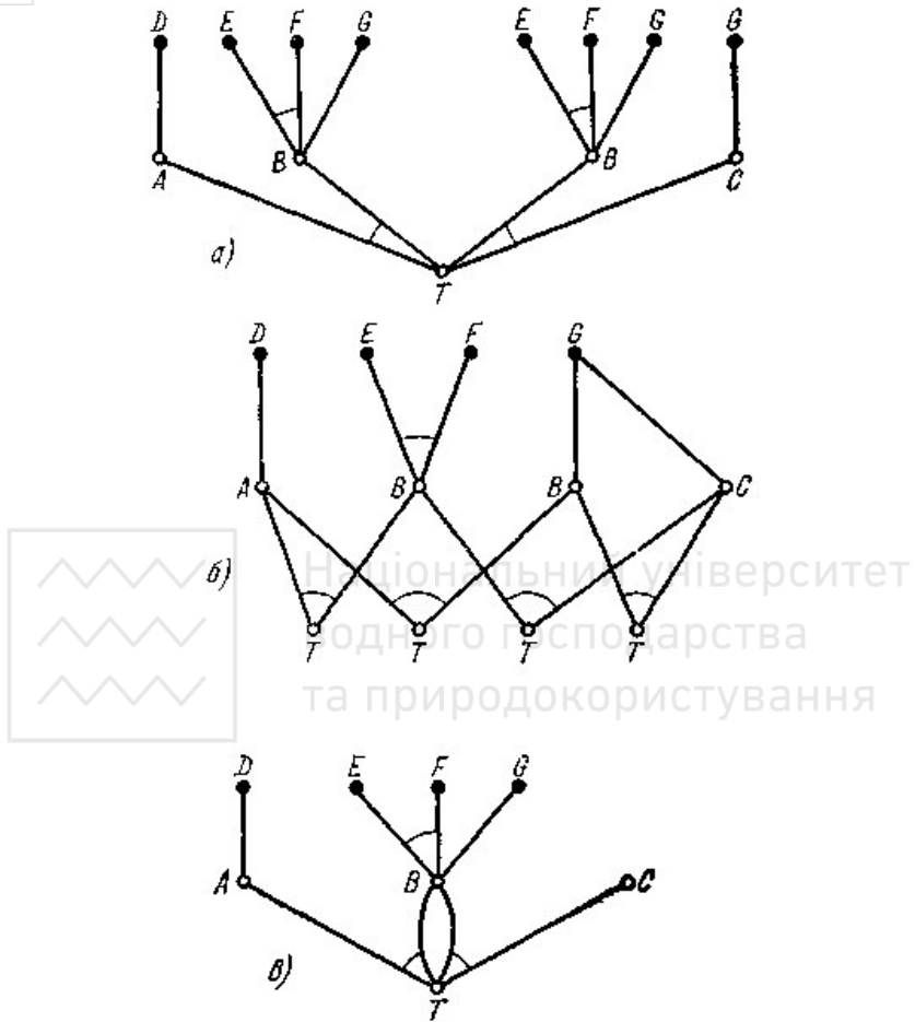
Рис. 10.10. Представление задачи T в виде пропозиционального дерева (а), графа доказательства определений (б) и графа вывода (в).
