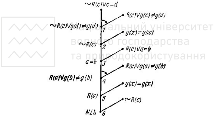
Рис. 12.7. Линейное опровержение с резольвацией и парамодуляцией.
