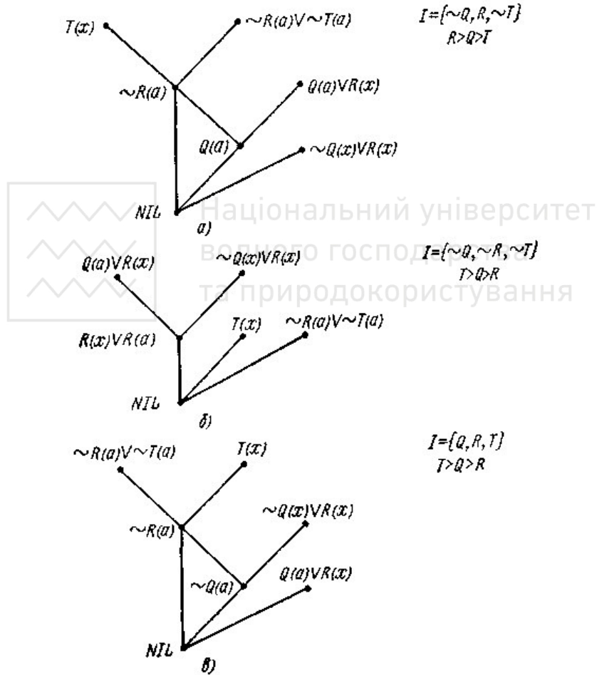
Рис. 12.2. Граф опровержения, полученный PI-резольвцией , положительной гиперрезольвцией и отрицательной гиперрезольвцией.
