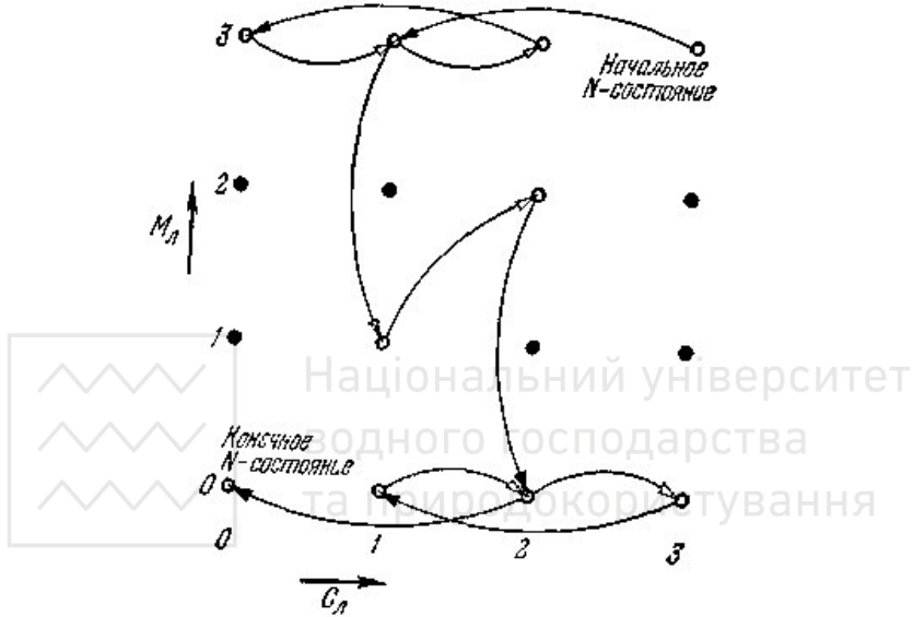
Рис. 10.2. Пространство N -состояний для элементарной задачи о миссионерах и людоедах.
