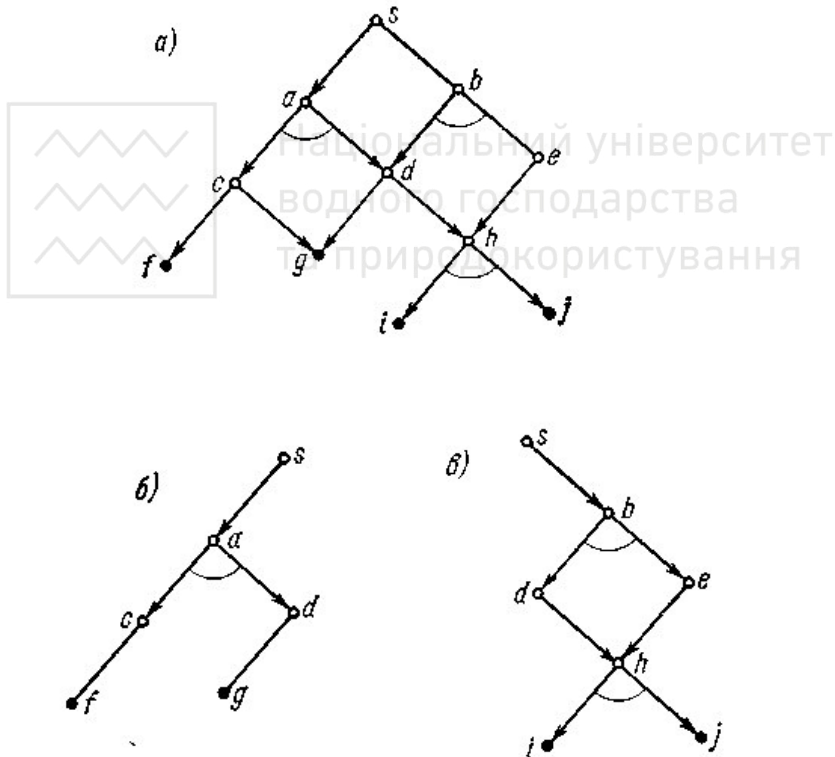
Рис. 4.4. Аддитивный пропозициональный граф ( a ) и его решающие графы ( б , в ).
