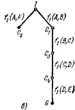
Рис. 10.11. Граф поиска пути из A в E (а) и соответствующий ему контекстный граф (б).
