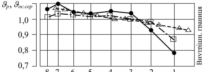
Рис. 3. Розрахункові й осереднені осьові швидкості у перерізі II-II (позначення аналогічні рис. 2)
