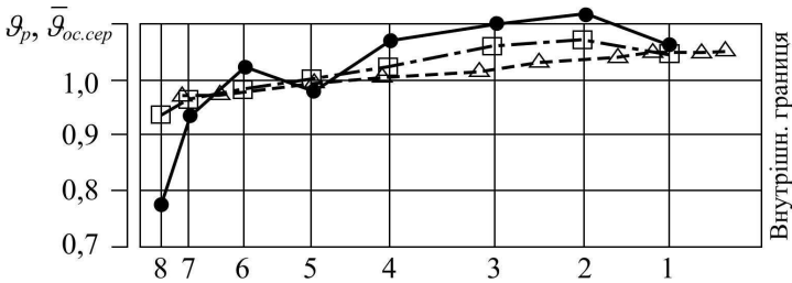
Рис. 4. Розрахункові й осереднені осьові швидкості у перерізі I-I (позначення аналогічні рис. 2)
