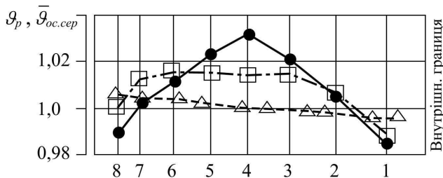
Рис. 2. Розрахункові й осереднені осьові швидкості у перерізі III-III: △ – результати розрахунку; ● – результати гідралічних досліджень; □ – результати досліджень на повітряному стенді
