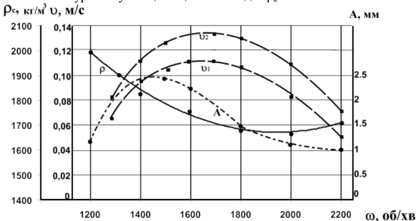
Рис. 1. Залежність густини середовища, швидкості спливання бурштину, амплітуди інтенсифікатора від частоти вібрації при експериментальних дослідженнях (A – амплітуда коливань вібронаряда; ρ – густина середовища; v_1 – швидкість спливання бурштину при подачі повітря q_{п} = 0,004 \text{ м}^3/\text{год.} ; v_2 – швидкість спливання бурштину при подачі повітря q_{п} = 0,006 \text{ м}^3/\text{год.} )
