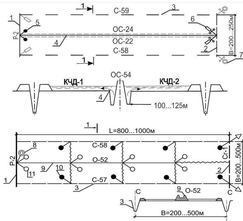
Рис. 2. Схеми карти-чека з дренажем (КЧД) та карти краснодарського типу (ККТ) Придунайських рисових систем
