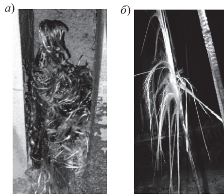
Рис. 3. Вигоряння полімерної матриці композитної арматури [14]: a – GFRP; б – CFRP.
