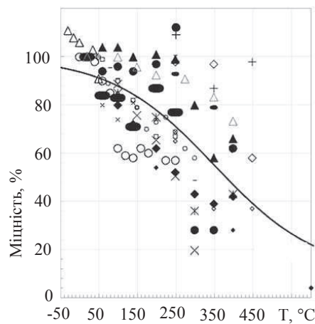
Рис. 4. Варіативність результатів експериментальних дослідів міцності CFRP та GFRP при підвищені температури [15].
