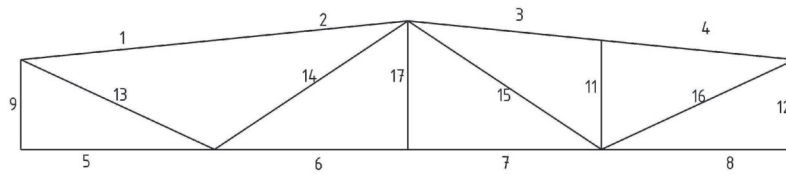
Схема ферми Ф-1 після руйнування стержня 14
