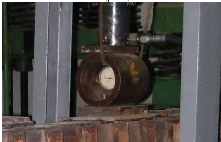
Рис. 3. Протарований кільцевий динамометр
