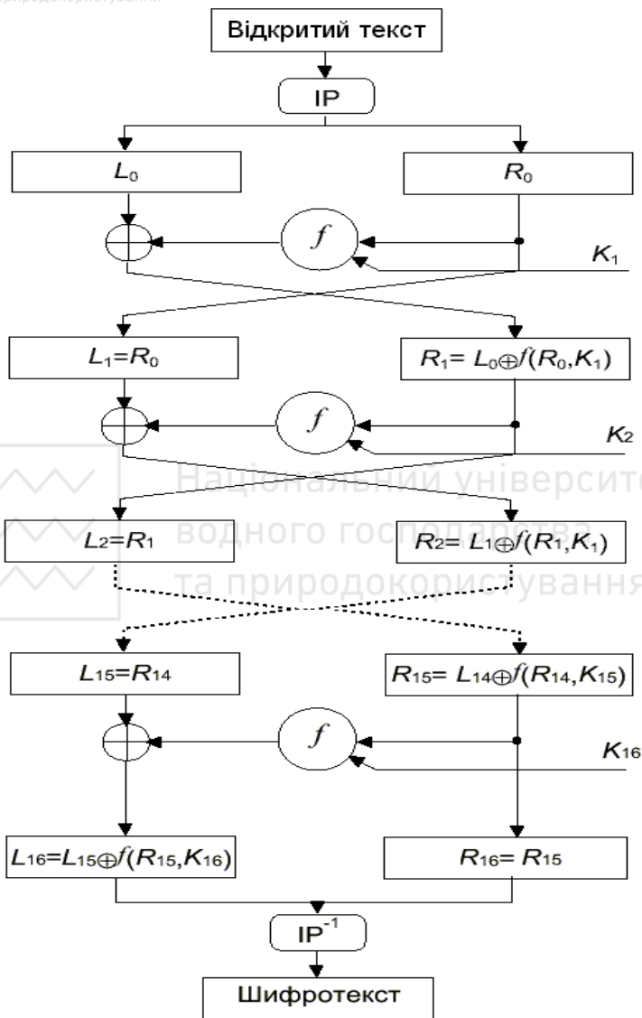
Рис 6. Схема перетворень блоку даних на етапах алгоритму DES
