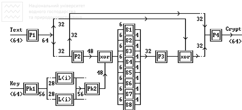
Рис.10 Блок-схема DES-алгоритму
