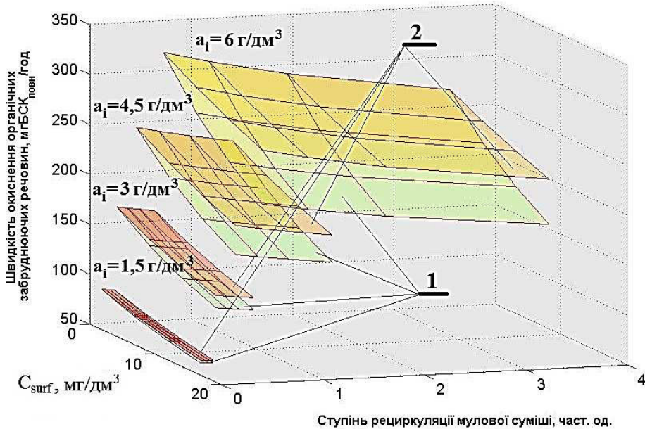
Рис. 4. Залежності швидкості окиснення органічних забруднюючих речовин в аеробних умовах від ступеня рециркуляції мулової суміші, дози мулу ( a_i , г/дм 3 ), початкової концентрації синтетичних детергентів ( C_{surf} , мг/дм 3 ) та ступеня їх біодеструкції: 1 – 0; 2 – 1
