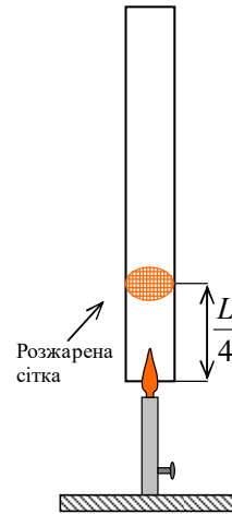
Рис. 2. Труба Рійке
