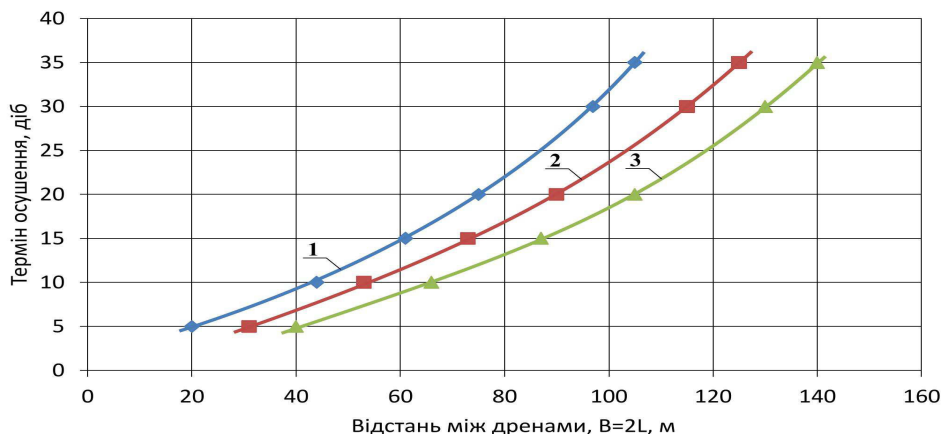
Рисунок. Залежність відстані між дренами від часу осушення ( h=1,5 м) рисового поля для умов Кілійської РЗС: 1 – без розпушення; 2 – несцільне розпушення; 3 – суцільне розпушення
