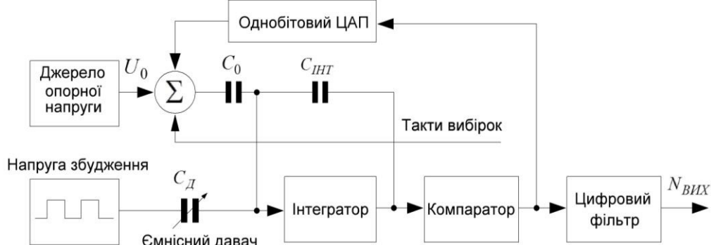
Рис. 3. Структурна схема сигма-дельта АЦП як вимірювача ємності
