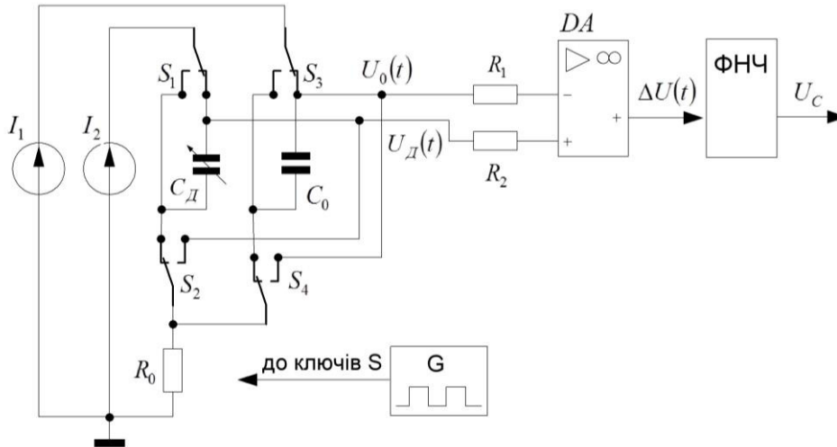
Рис. 6. Пояснення принципу перетворення відносного приросту ємності від номіналу на базі двох інтеграторів
