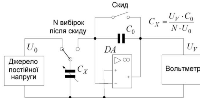
Рис. 1. До методу вимірювання ємності, основого на використанні зарядового підсилювача
